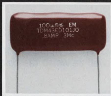
Typical TDM43 Capacitor, actual size
