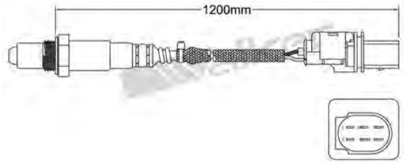
800-95006 AUDI 2004-2009 / VOLKSWAGEN 2004-2010 Linear Wideband Sensor
