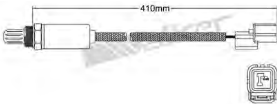
250-21031 HONDA 1995-2001 Unheated Lambda Sensor
