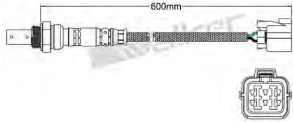
250-54047 SUBARU 2005-2007 Air/Fuel Ratio Sensor
