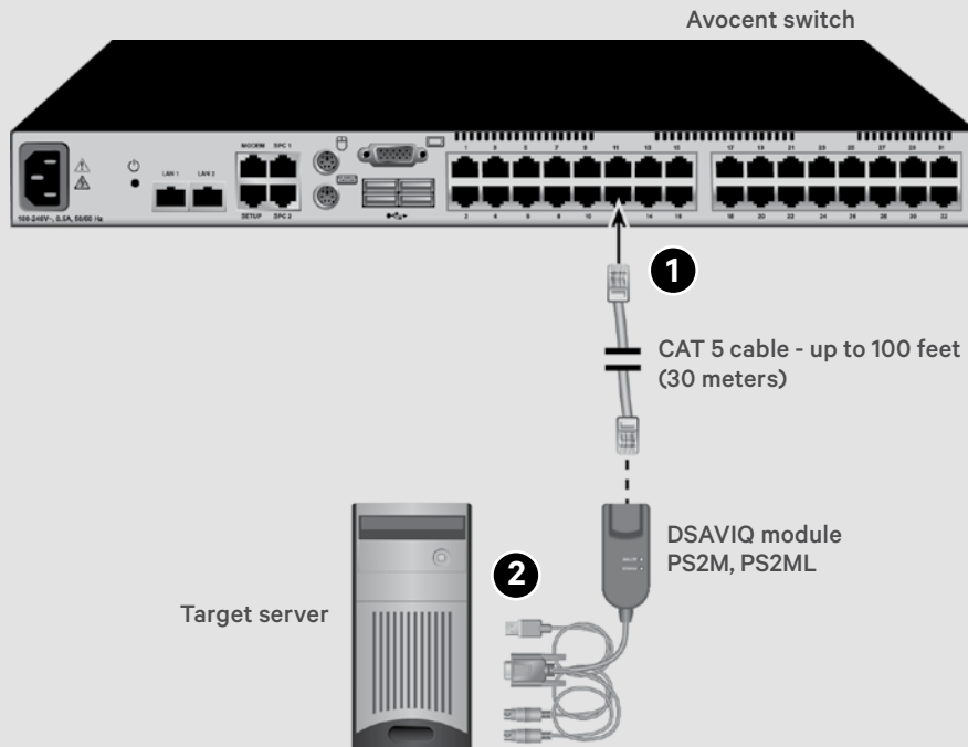
DSAVIQ-PS2M module configuration
