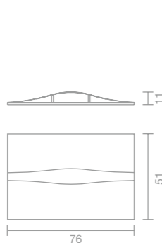
ART. 4500 Applique / Wall lamp Applique / Wandleuchte
