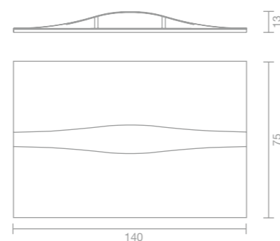
ART. 4501 Applique / Wall lamp Applique / Wandleuchte
