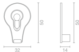
ART. 2745 Applique / Wall lamp Applique / Wandleuchte
