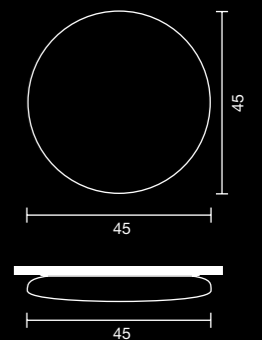
ART. 2421 Plafoniera / Ceiling lamp Plafonnier / Deckenleuchte
