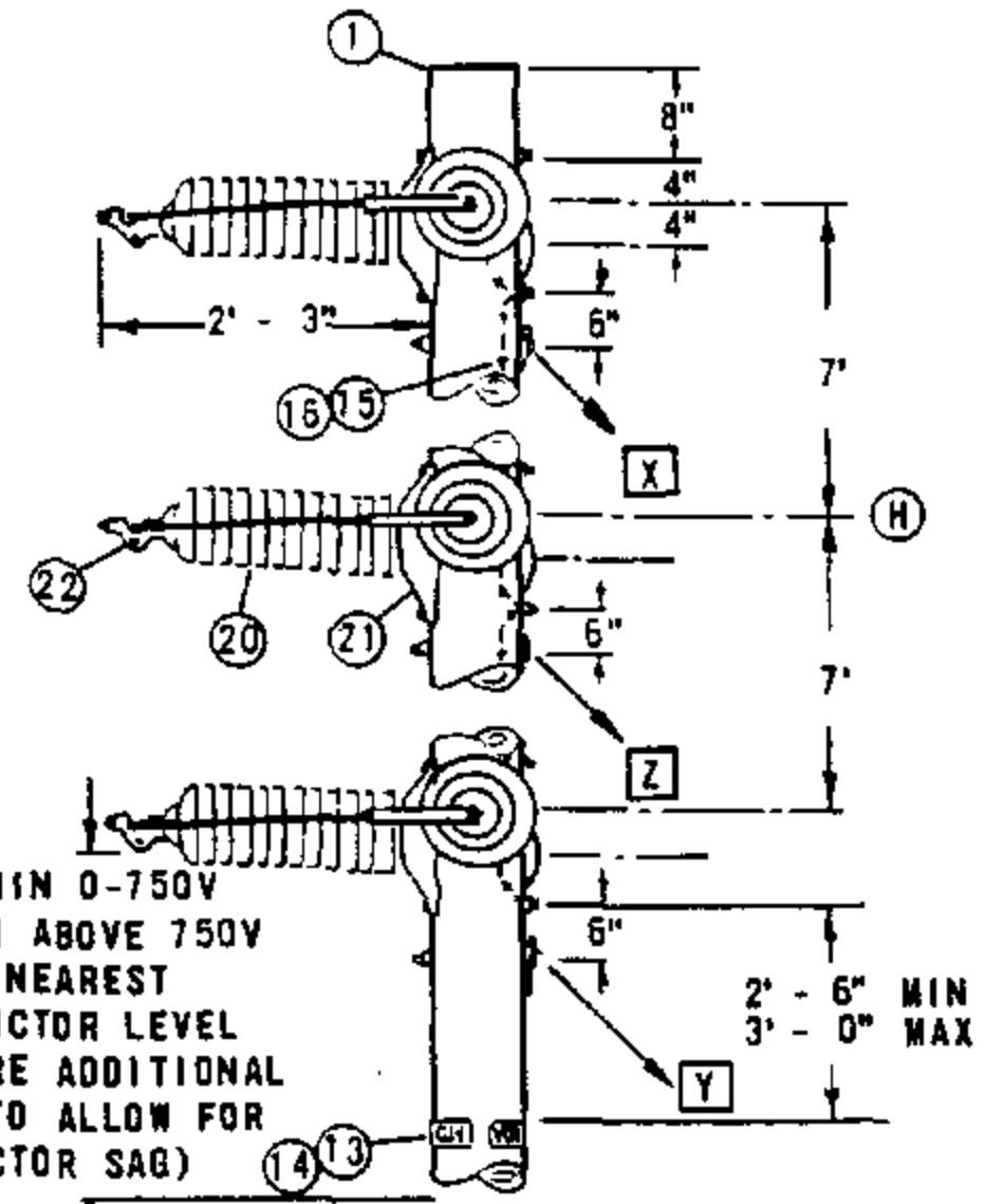
ELEVATION
