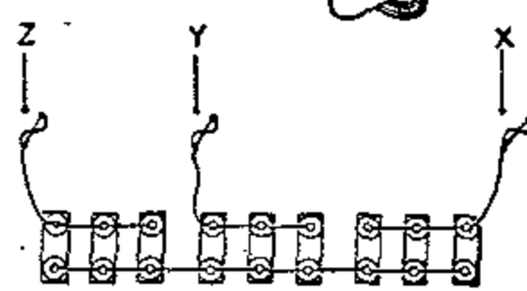
DIAGRAM OF 12KV WYE CONNECTIONS 900 KVAR (9-100 KVAR UNITS) 450 KVAR (9-50 KVAR UNITS) 225 KVAR (9-25 KVAR UNITS)
