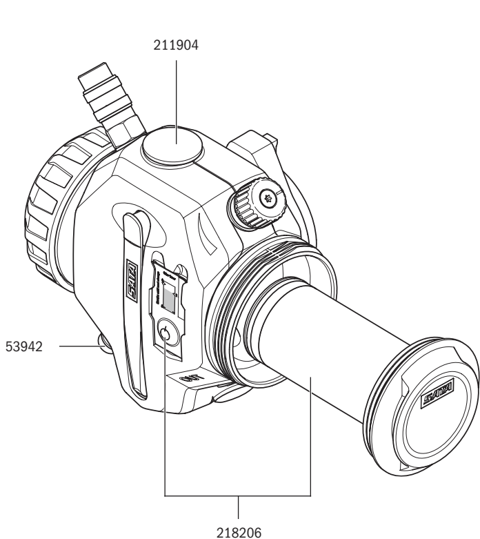
SATA air carbon regulator Art. Nr. 1000182
