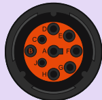
Pin assignment DEUTSCH Type 1
