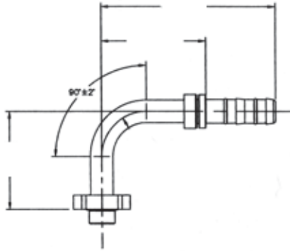
90° Pad Style Connection ( olvo)
