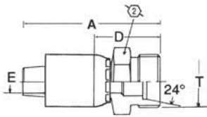
Male DIN 24° Seat I.Rh (Light)
