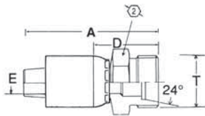
Male DIN 24° Seat s.Rh (Heavy)
