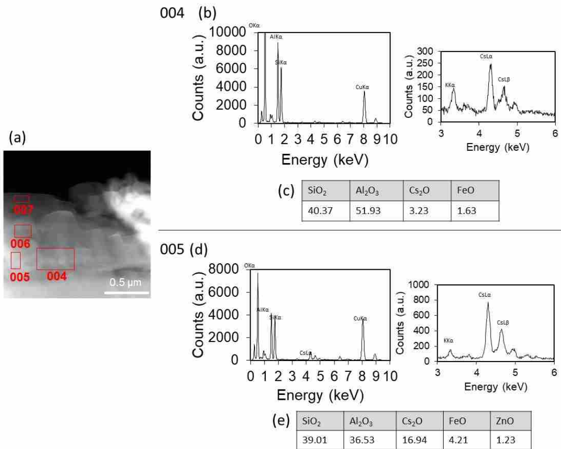
図 I -2-2-3-17 放射性粒子 D1-MAX の(a)STEM 撮影画像。STEM-EDX による面分析範囲 004 の (b)EDX スペクトルおよび(c)スペクトルから計算した化学組成の定量結果(重量%)。STEM-EDX による面分析範囲 005 の (d)EDX スペクトルおよび(e)スペクトルから計算した化学組成の定量結果(重量%)。面分析範囲を赤色の枠で示す。
