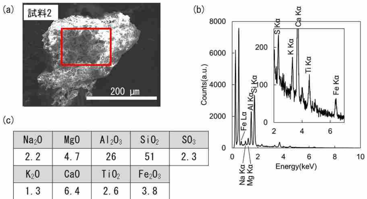
図 I -2-2-3-22 SEM-EDX による放射性粒子 D1-MID (試料 2)の(a)面分析範囲、(b)面分析範囲における EDX スペクトルおよび(c)スペクトルから計算した化学組成の定量結果(重量%)。面分析範囲を赤枠で示す。
