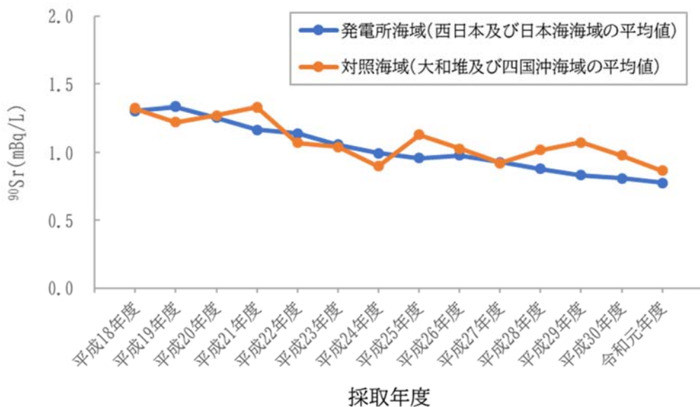
図 I -2-1-1-5 対照、西日本及び日本海海域で採取した表層海水に含まれる ^{137}\text{Cs} と ^{90}\text{Sr} の放射能濃度の平均値を経年変化として示したもの（上図 ^{137}\text{Cs} ; 下図 ^{90}\text{Sr} ）
