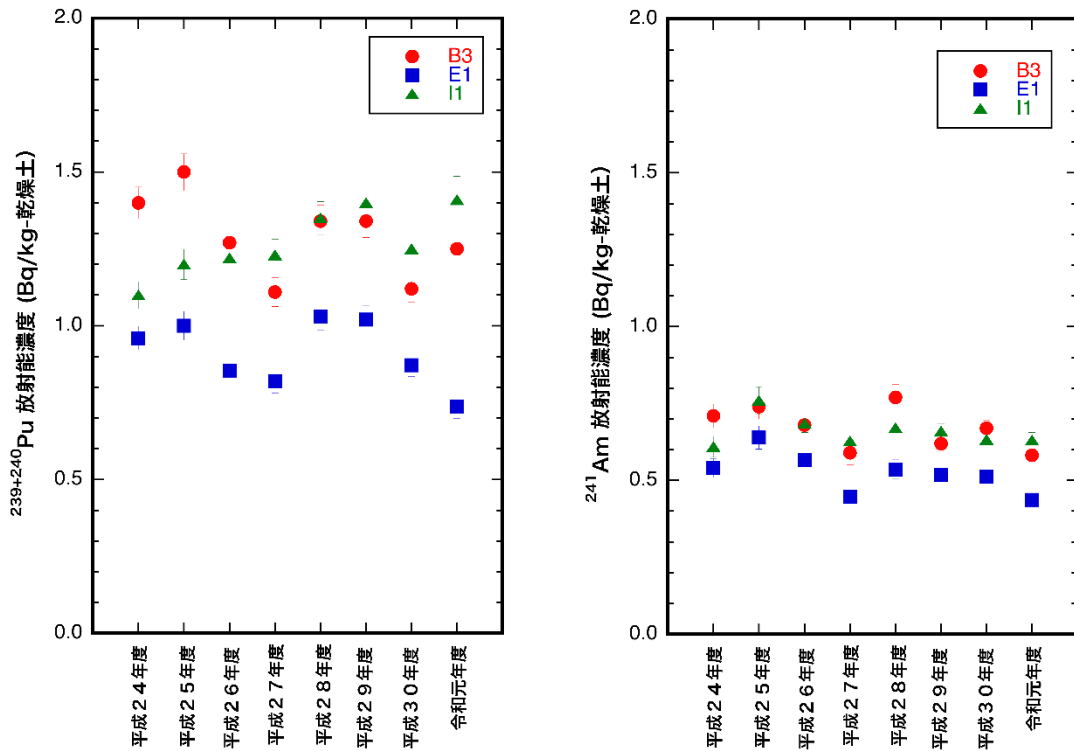
図II-3-22 各測点で採取した海底土試料に含まれる ^{239+240}\text{Pu} と ^{241}\text{Am} の放射能濃度の平成24年度から平成31（令和元）年度の時系列変化
