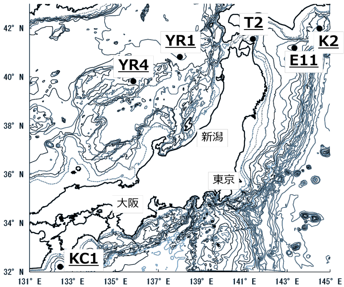
図 I -2-1-1-1 対照海域における調査測点。襟裳沖海域（襟裳沖：E11、核燃料沖：T2、釧路沖：K2）、大和堆海域（YR1、YR4）及び四国沖海域（KC1）
