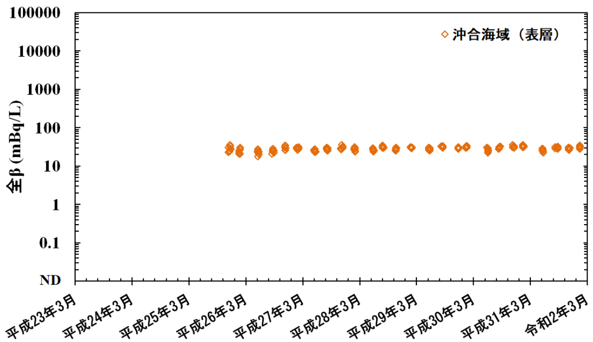
図 II-3-9 沖合海域で採取した海水試料に含まれる全ベータ放射能の時系列変化
