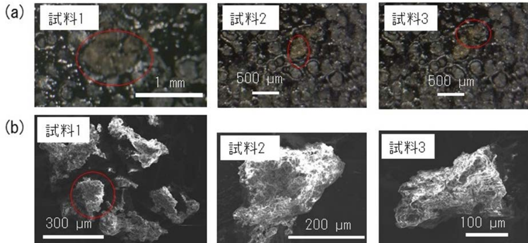
図 I-2-2-3-20 放射性粒子 D1-MID の(a)実体顕微鏡により撮影した画像、(b)SEM による撮影画像。
