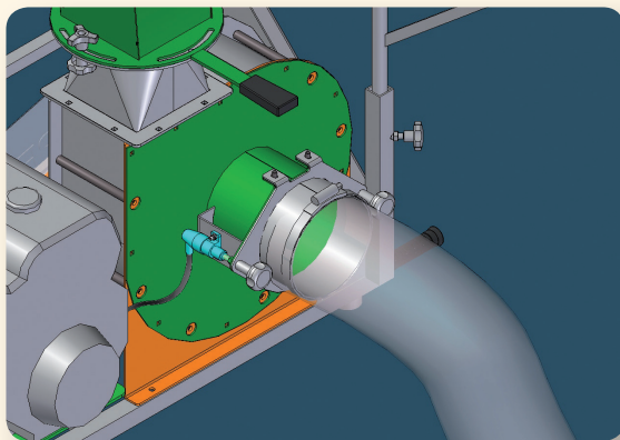
Dispositivo di sicurezza blocco motore Engine stop safety device Dispositif de sécurité de bloquage moteur Sicherheit Klemme für Motor
