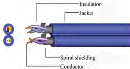
DX0022A EKG raw cable
