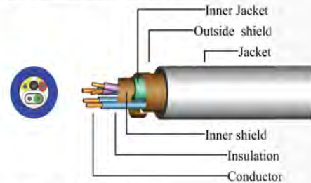
DX0009A ECG raw cable
