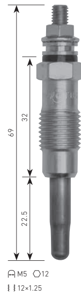
B-078 MERCEDES-BENZ OM 601.912, etc. ⚡11.5V
