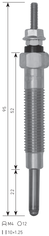
PM-75 MITSUBISHI 4D55, 4D56 ⚡12V
