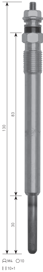
B-112 MERCEDES-BENZ OM 668 ⚡11.5V
