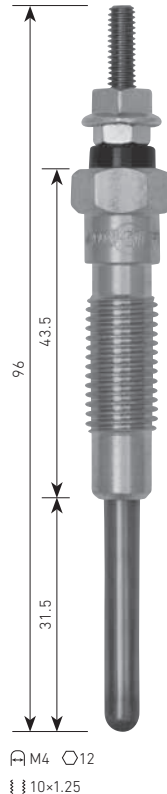
PT-144 TOYOTA L 411V
