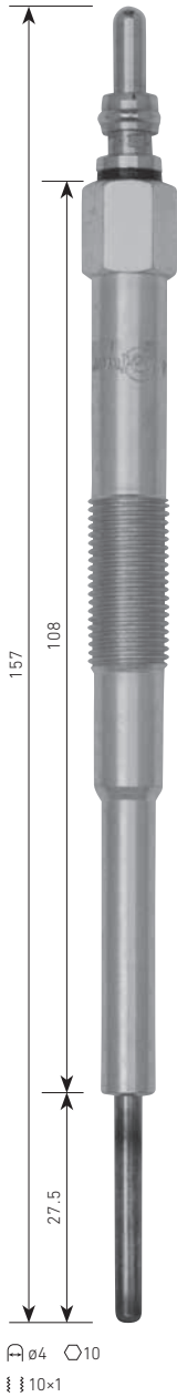
PR-801 SUBARU EE20Z ⚡11V
