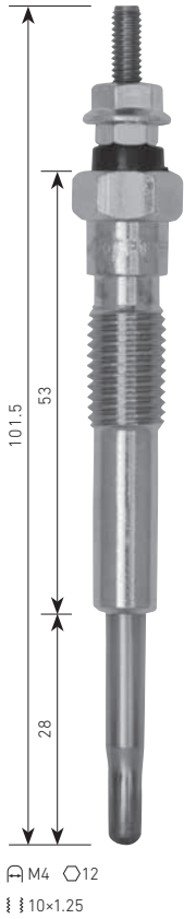
PT-158 TOYOTA 1HZ ⚡11V
