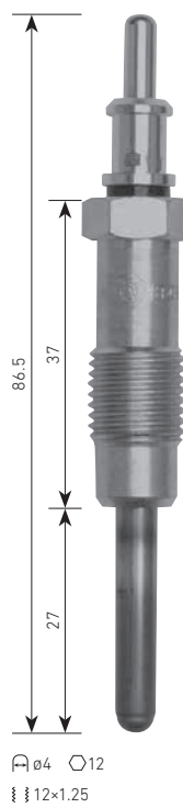
B-067 MERCEDES-BENZ OM 602.980 ⚡11.5V
