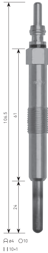
B-118 LAND ROVER 10P, 14P, 15P ⚡11V
