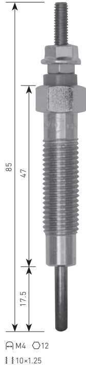
CP-07 MITSUBISHI 4D56T, etc. ⚡11V
