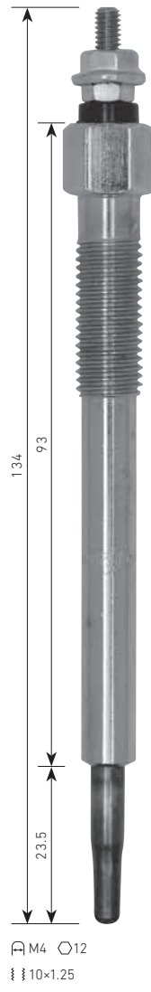
CP-52 RENAULT ⚡11V
