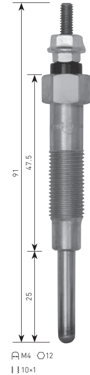
PN-126 NISSAN CD17 ⚡6.5V
