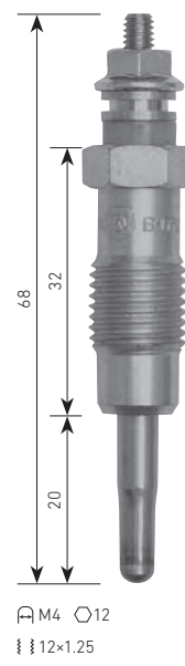
B-072 CITROËN K9A (TUD3), K9Y (TUD3Y) ⚡11.5V
