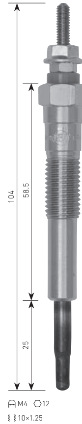
CP-22 TOYOTA 1KZ-TE, etc. ⚡11V
