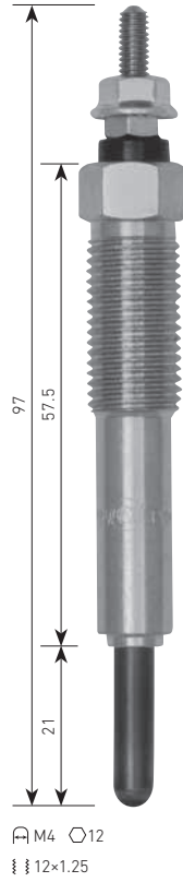
PM-160 MITSUBISHI 4D30 ↖24V
