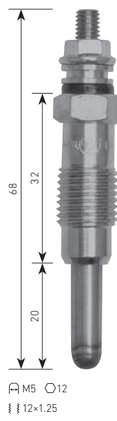
B-053 FORD LTA, LTB, LTC ⚡11.5V
