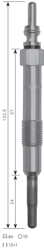
B-109 FIAT 182 B4.000, etc. 11V
