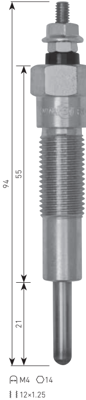
PN-125 NISSAN ED33 ⚡23V
