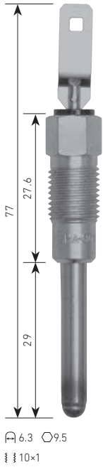
PA-306 CHEVROLET L56 ⚡10.5V
