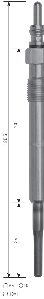
B-111 AUDI AFB, etc. 11V
