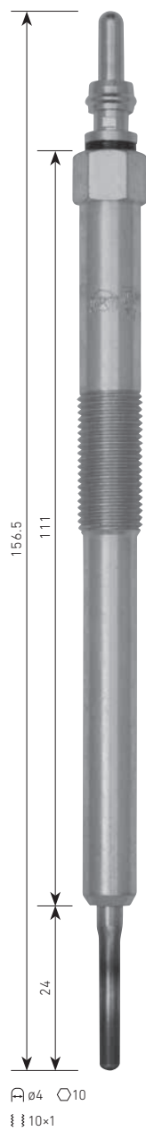
A-609 SSANGYONG D27DTP ⚡5V
