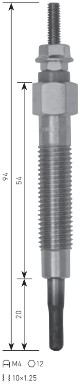
CP-06 MITSUBISHI 4D56, etc. ⚡11V
