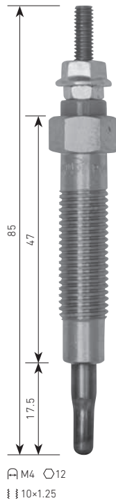
PM-167 MITSUBISHI 4D56T, 4D68 ↖11V
