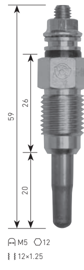
B-080 RENAULT F8Q ⚡11V
