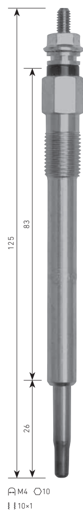
B-074 LAND ROVER 23L, etc. ⚡11.5V
