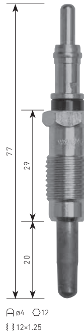
B-119 FIAT 188 A3.000, etc. ⚡11V
