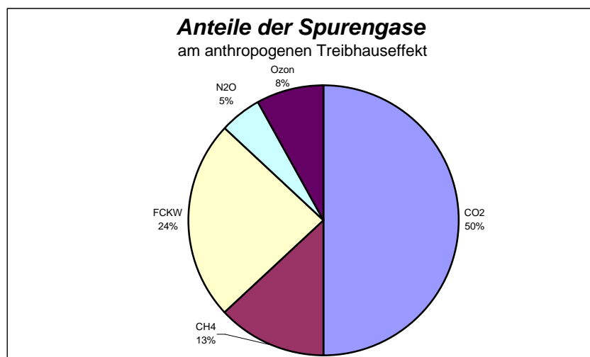
Abbildung 10-2 Anteile der Spurengase
