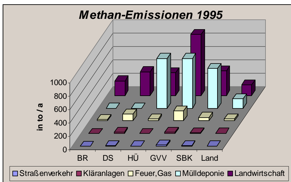
Abbildung 10-4 Methan Emissionen 1995
