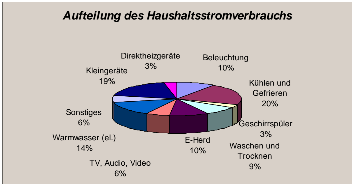
Abbildung 17-5 Aufteilung Haushaltsstromverbrauch
