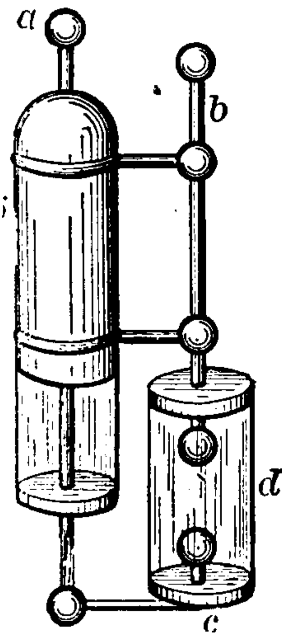
Fig. 315. Unit Jar.
