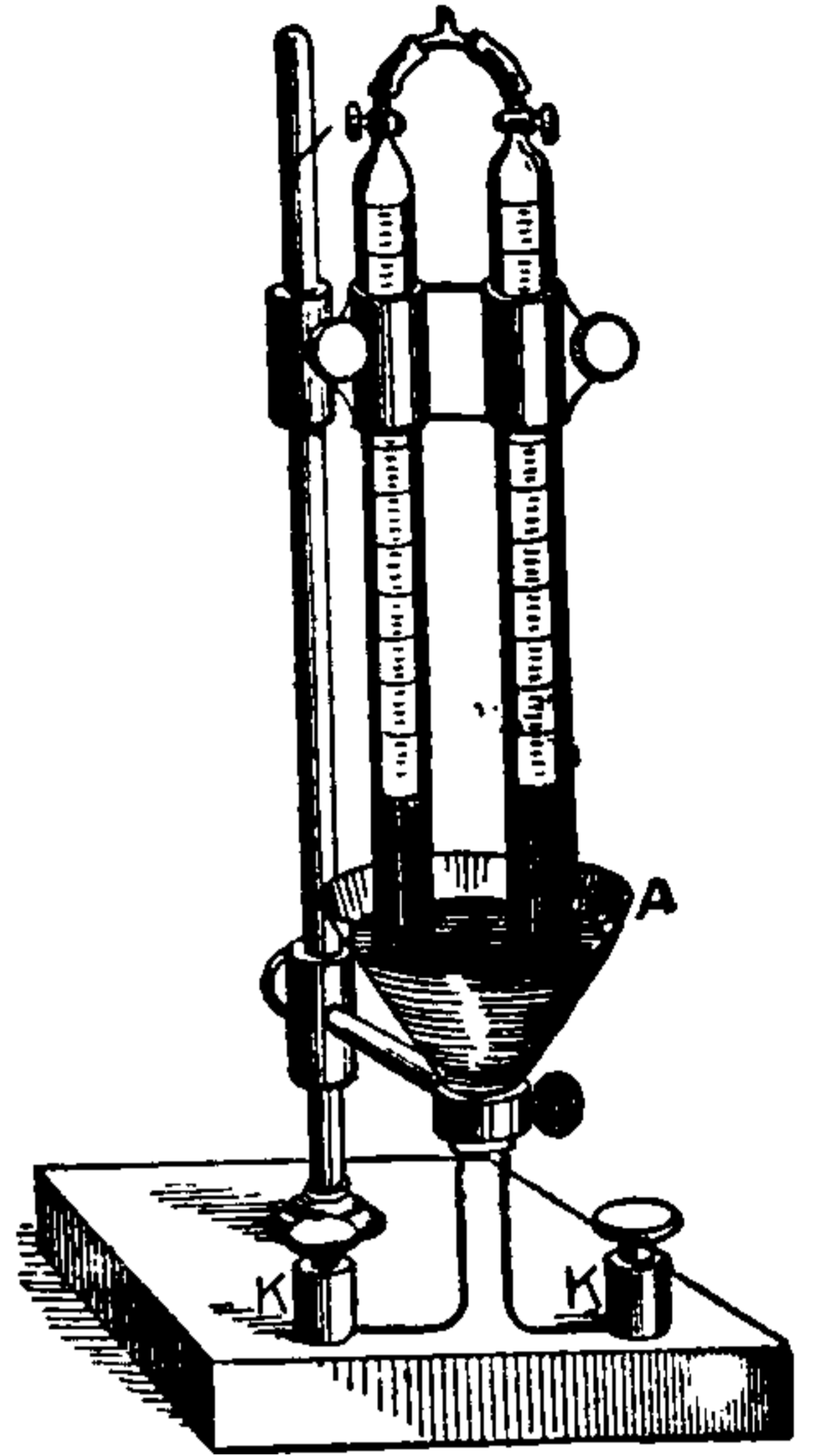
Fig. 241. Eudiometer.
