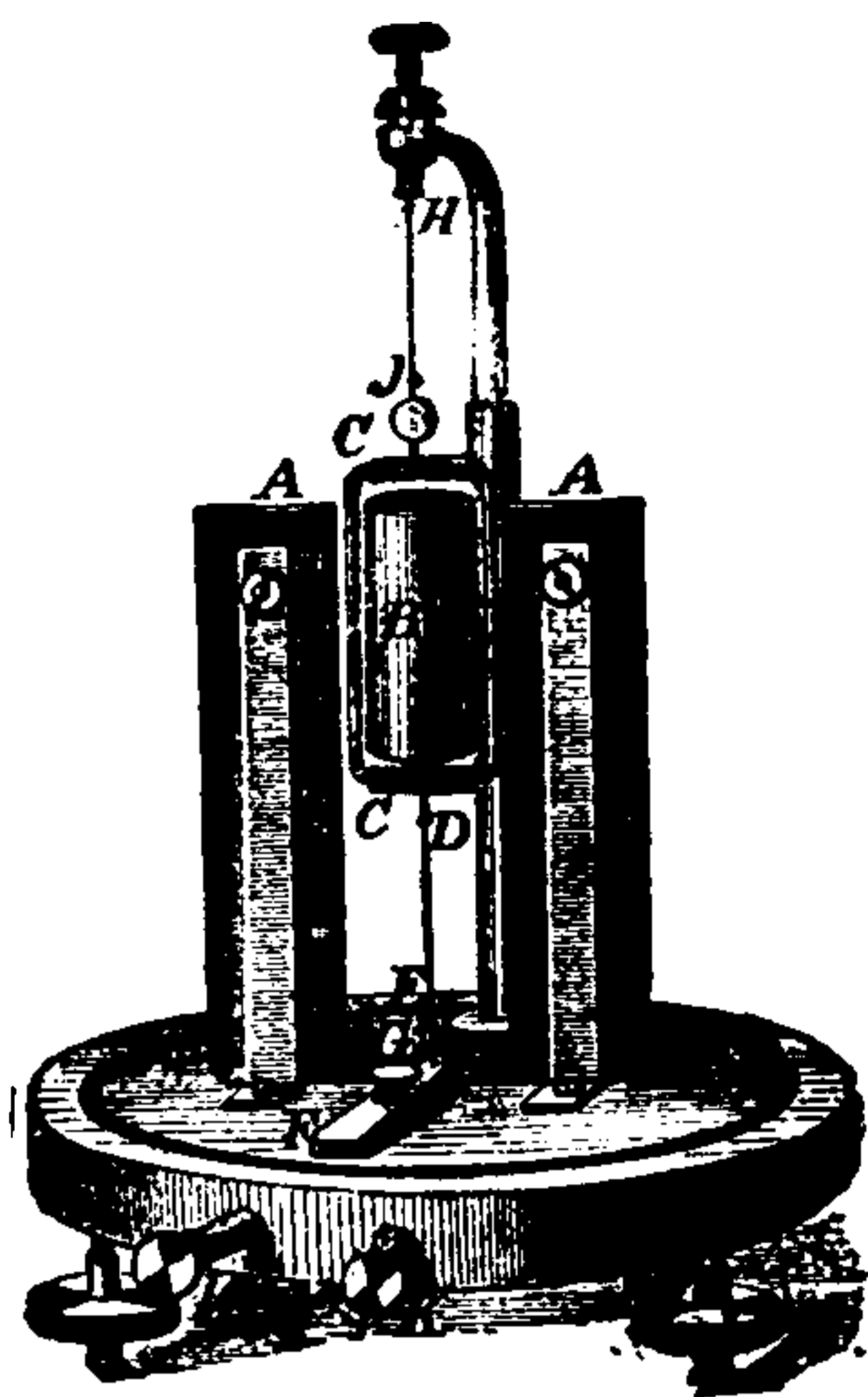
Fig. 271. Deprez-D'Arsonval Galvanometer.
