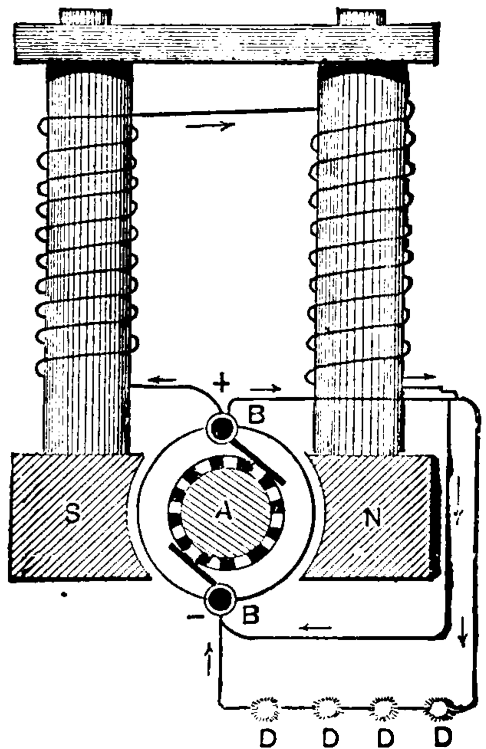
Fig. 357. Shunt Dynamo.
