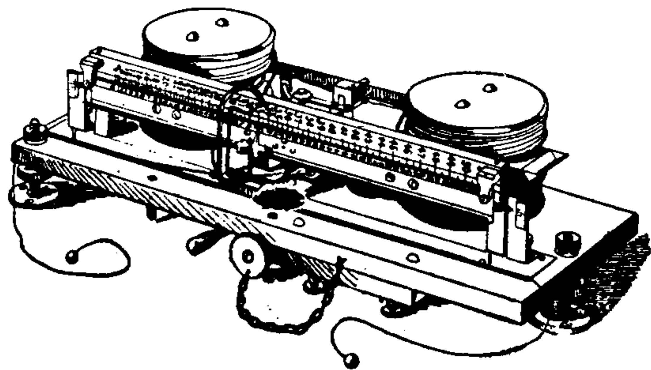
Fig. 33. Centi-Ampère Balance.
