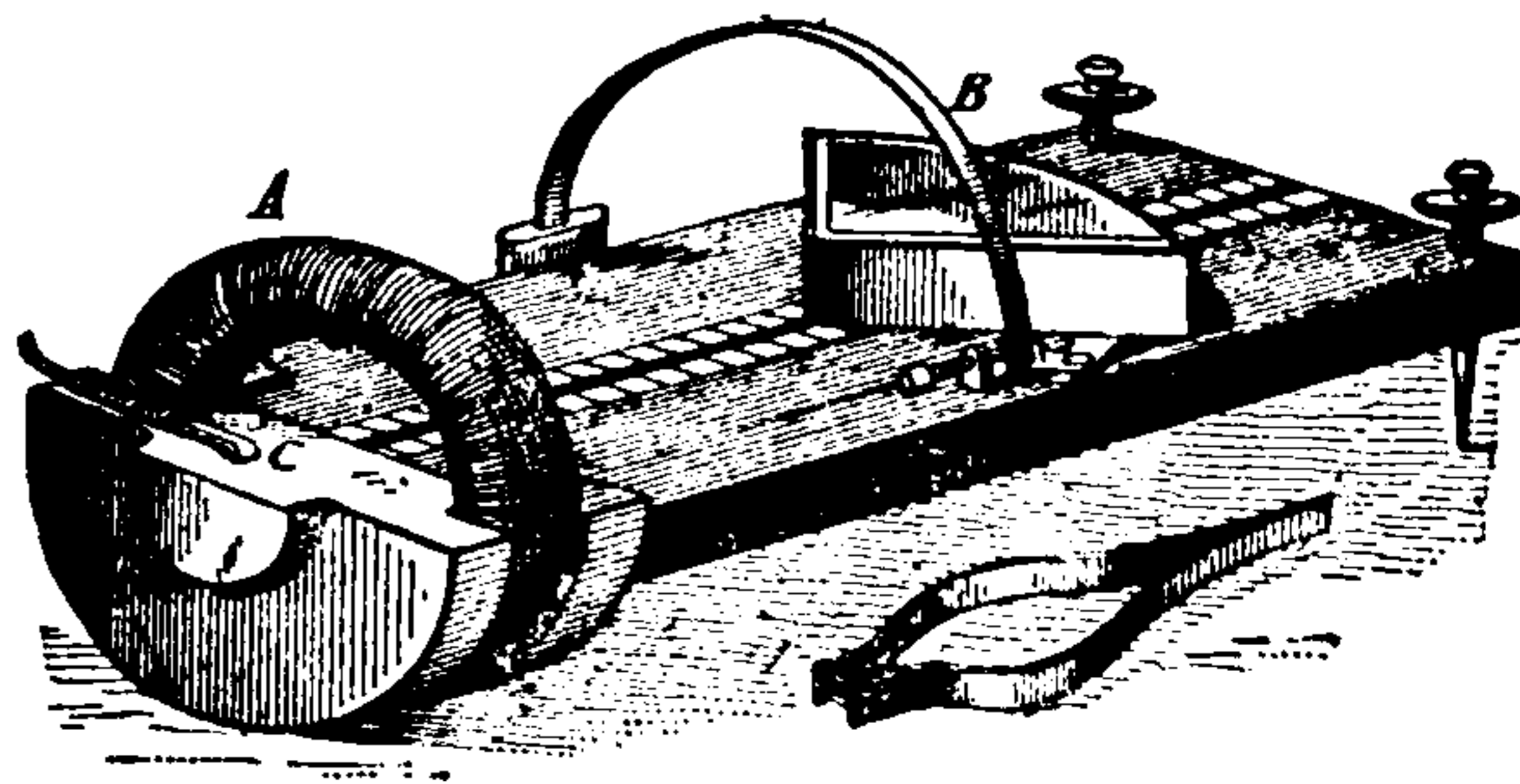
Fig. 280. Galvanometer Voltmeter.
