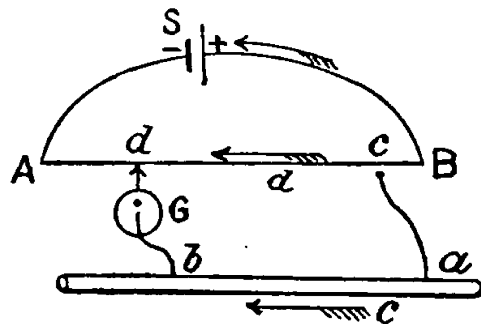
Fig. 451. Potentiometer.
