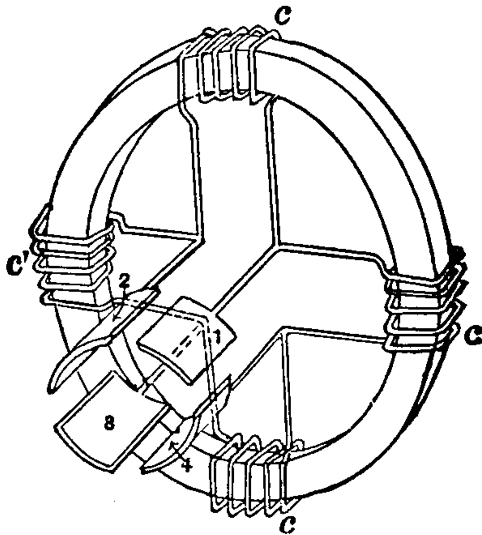
Fig. 23. Ring-Armature.
