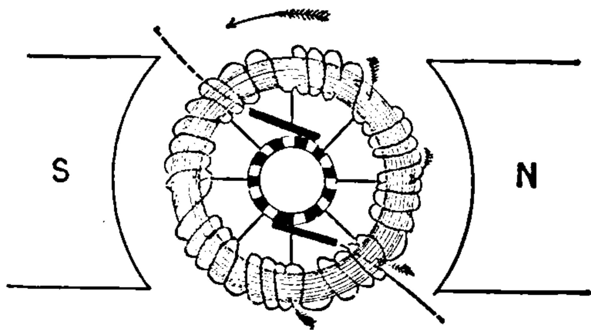
Fig. 20. Bi-polar Armature.
