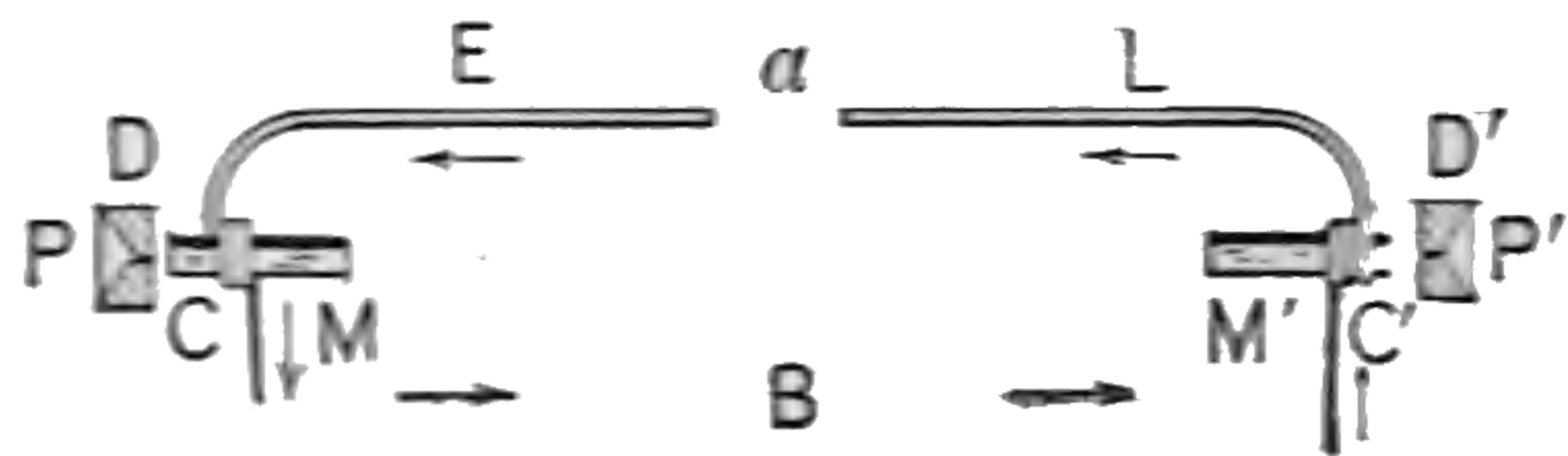
Fig. 550. Telephone Circuit.
