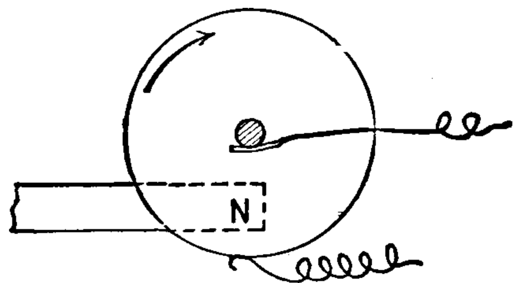
Fig. 204. Faraday's Disc.
