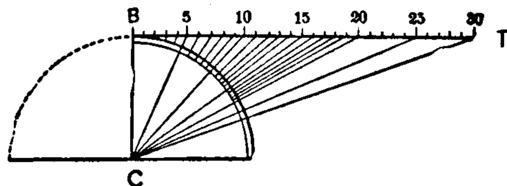
Fig. 497. Tangent Scale.
