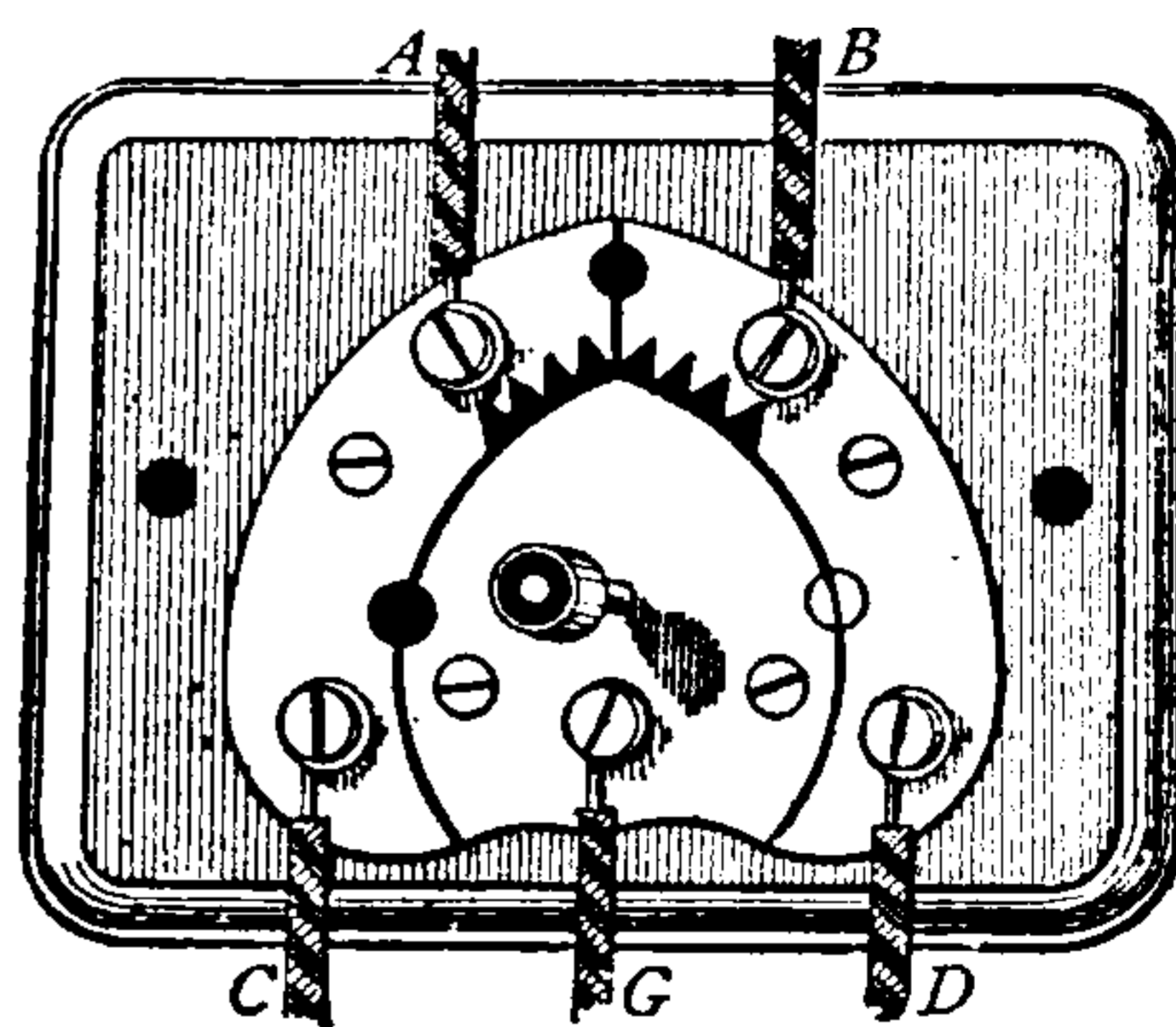
Fig. 25. Comb Lightning-Arrester.
