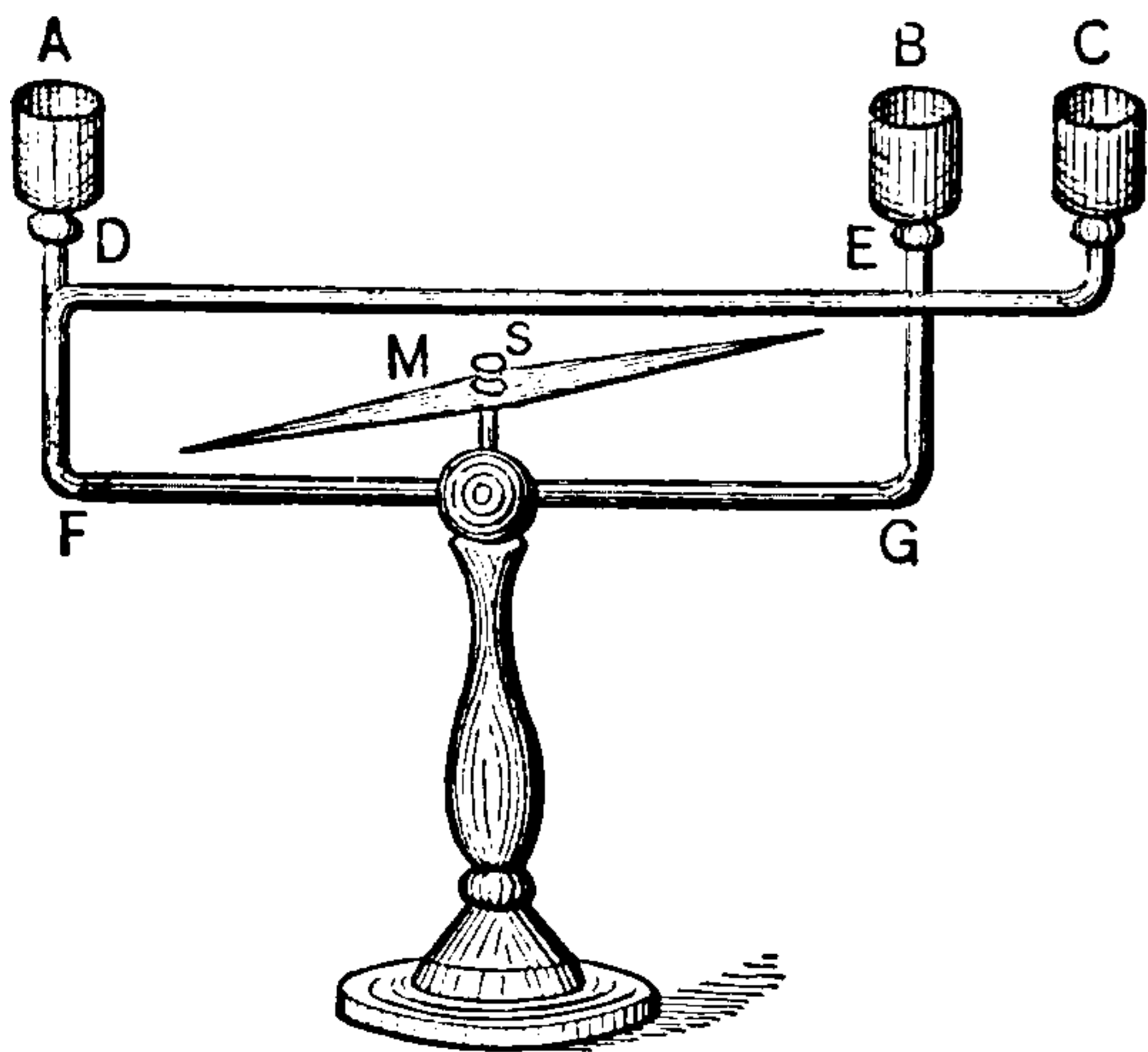
Fig. 265. Ampère's Apparatus.
