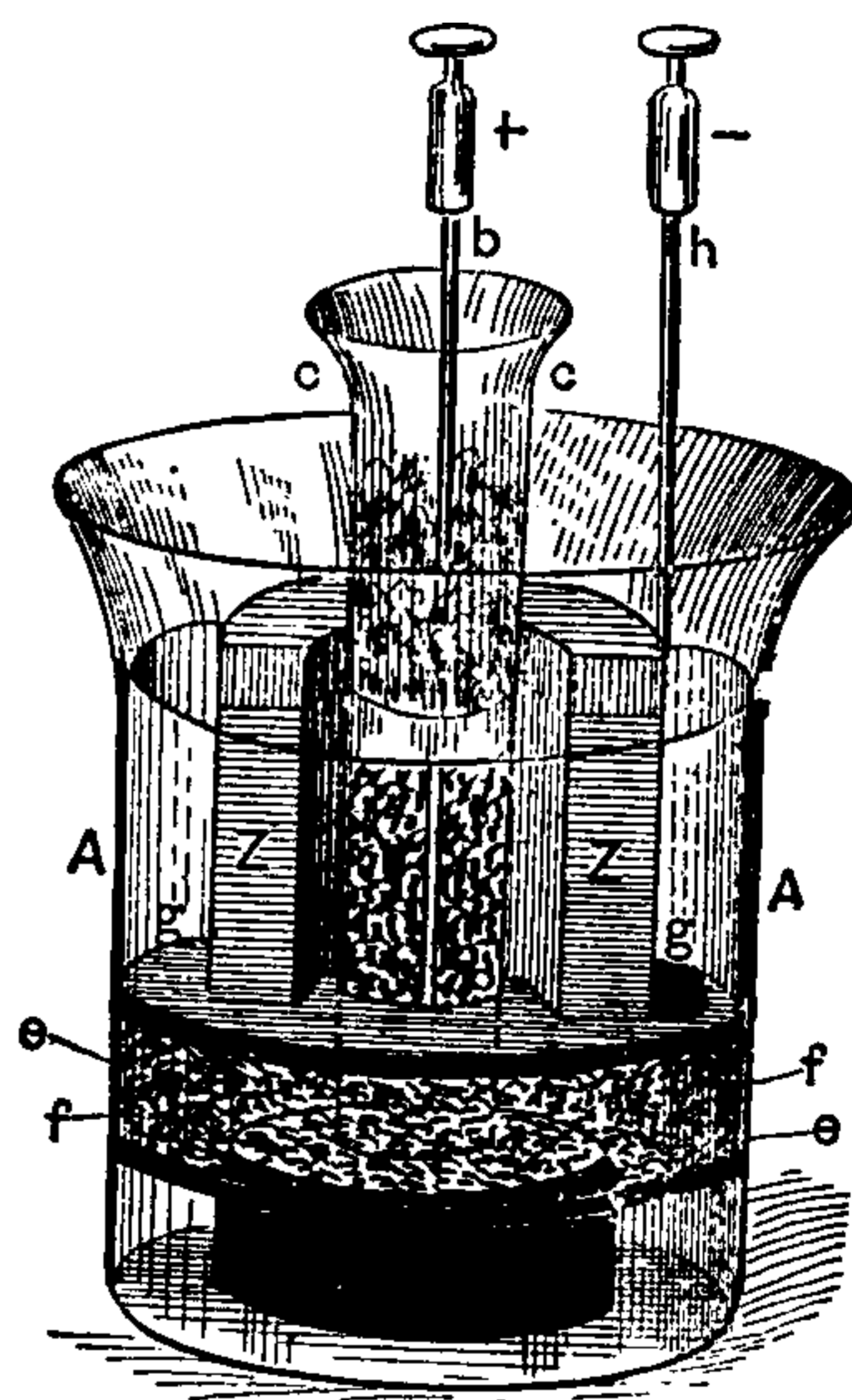
Fig. 113. Siemens-Halske Cell.
