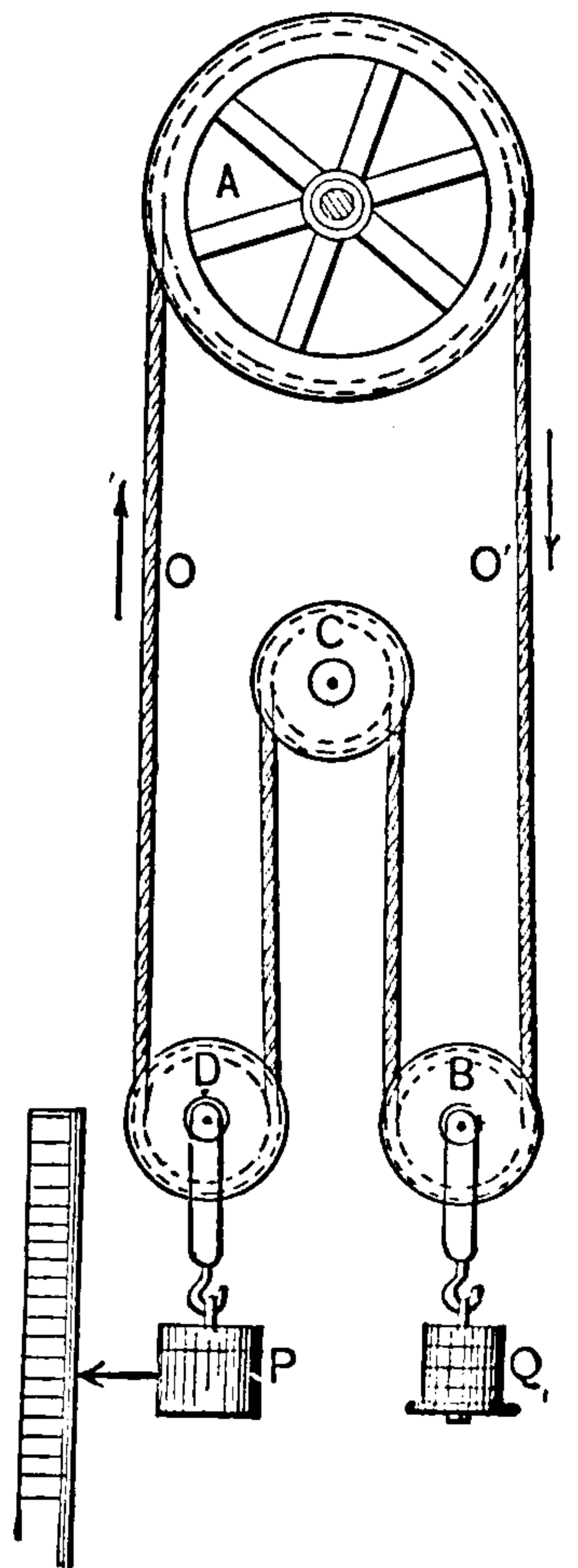
Fig. 223. Parsons' Dynamometer.
