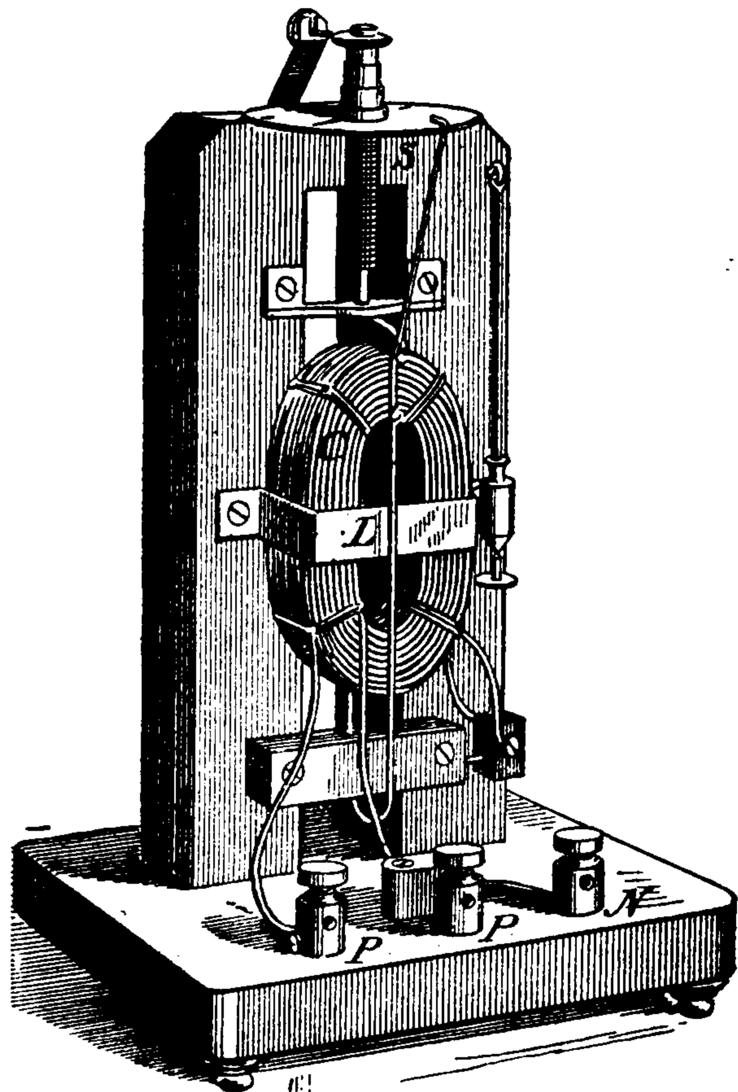
Fig. 224. Siemens' Electro-Dynamometer.
