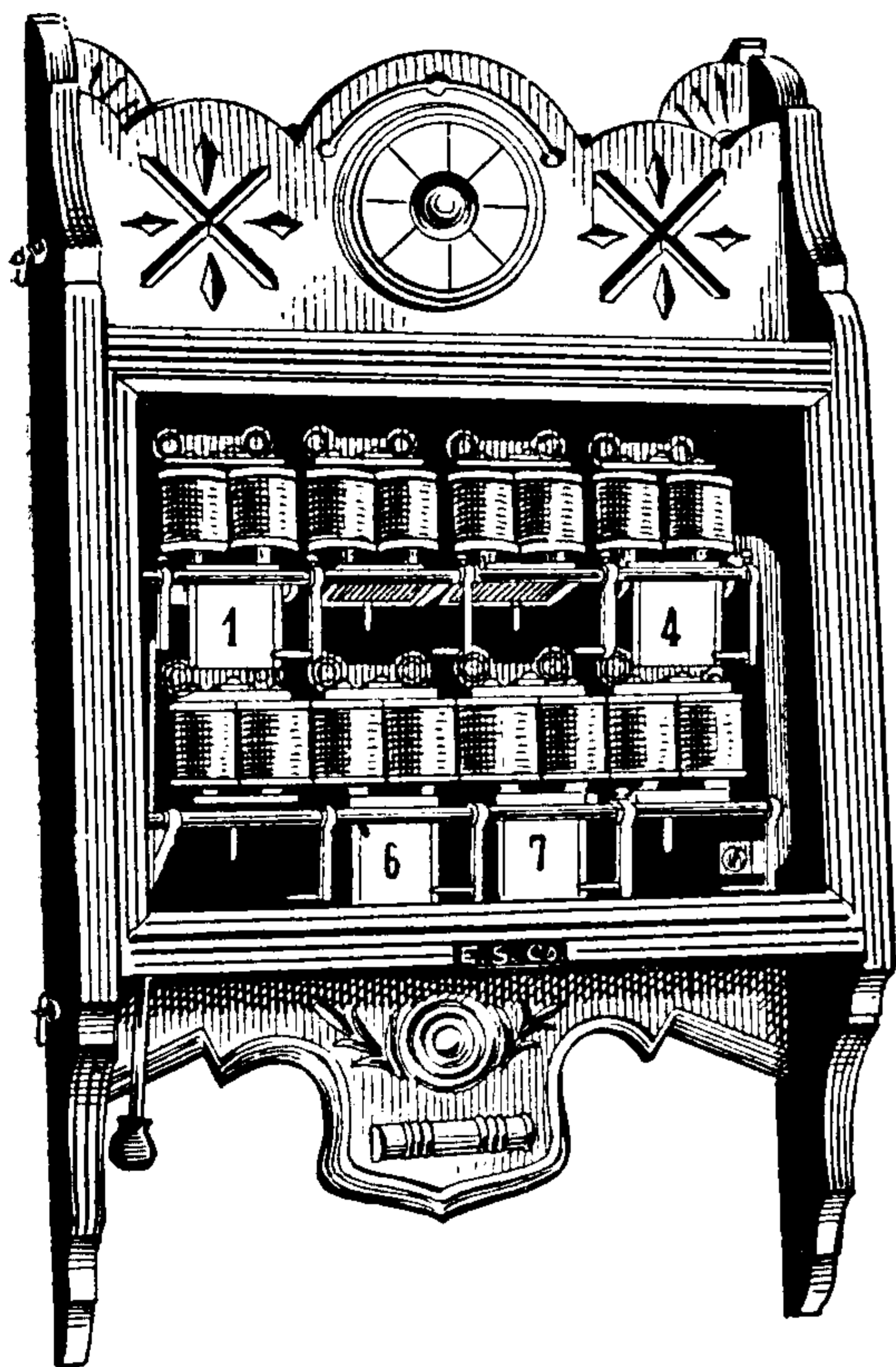
Fig. 16. Gravity-Drop Annunciator.
