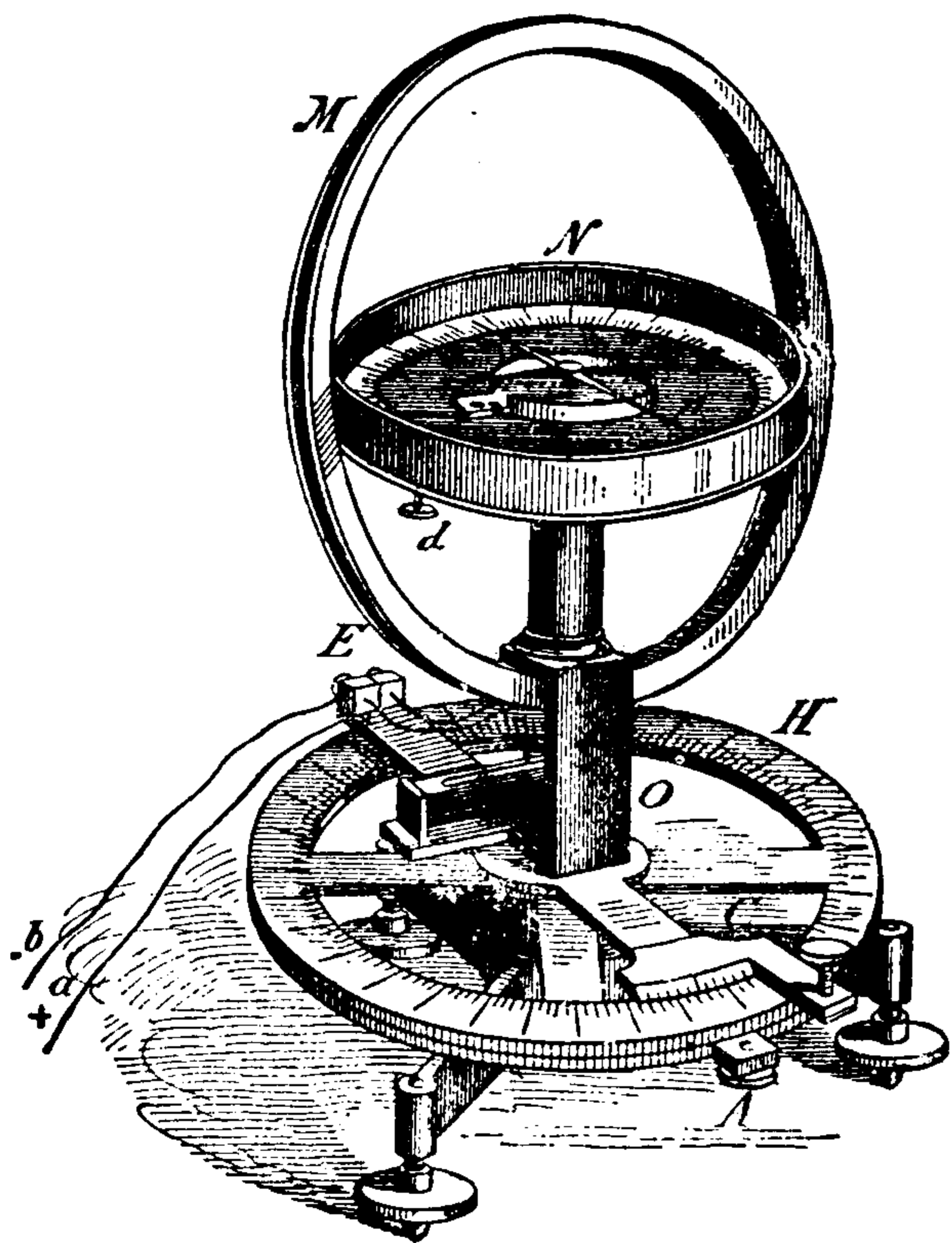
Fig. 276. Sine Galvanometer.
