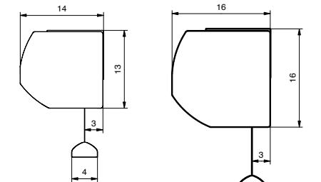
Profil petit carter alimentation à droite
