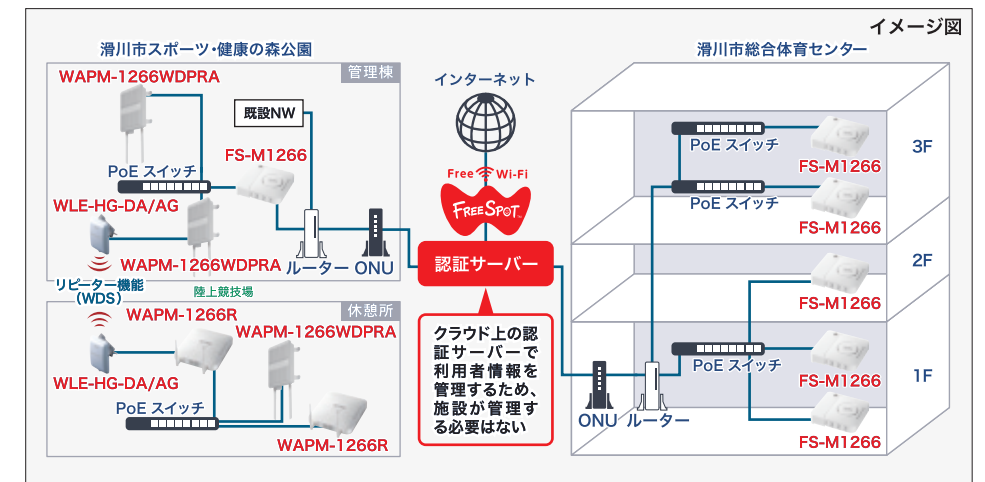
滑川市総合体育センターには、緊急モードに対応している「FREESPOT」導入キット「FS-M1266」を設置。滑川市スポーツ・健康の森公園の管理棟と休憩所周辺は屋外対応モデル「WAPM-1266WDPRA」をそれぞれ設置。
