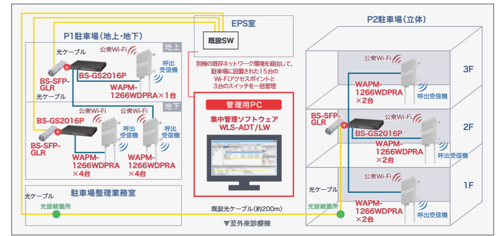
機器設置後の運用・メンテナンス性、また、屋外設置が必要な環境条件を加味してWi-Fiアクセスポイントは「WAPM-1266WDPRA」で統一。約200m離れているP1・P2駐車場の接続には光ケーブルと光トランシーバーを採用することで、通信速度・安定性を確保しつつ管理工数の削減も実現。
