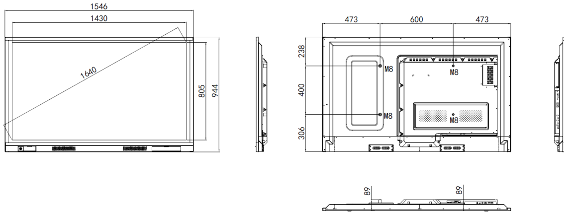
AVE-6510 Dimensions
