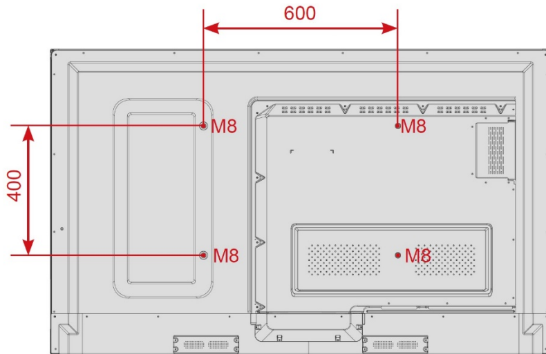
AVE-6510
