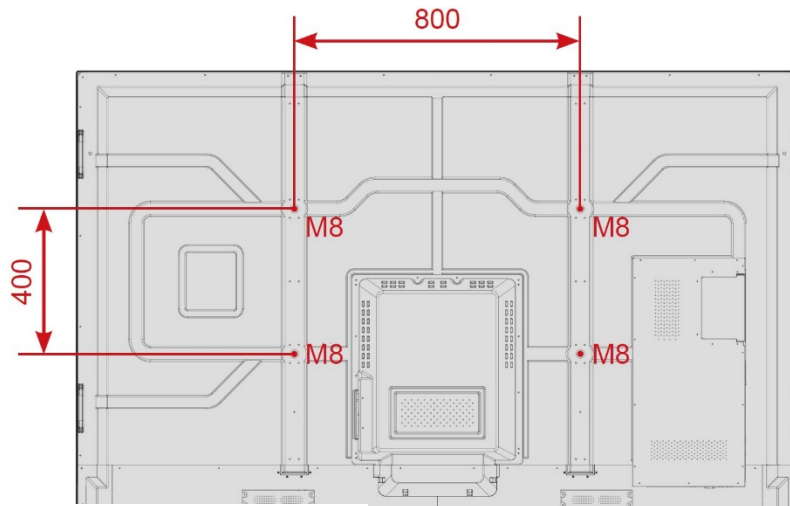
AVE-7510 / 8610
