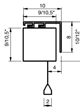
Schéma de profil - Moteur à droite.
