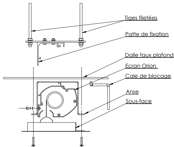
Principe de la sous-face
