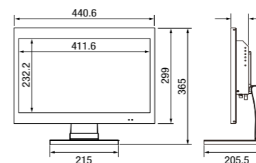
外形寸法図 (mm)
