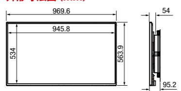
外形寸法図 (mm)
