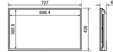
外形寸法図 (mm)
