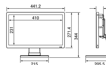
外形寸法図 (mm)
