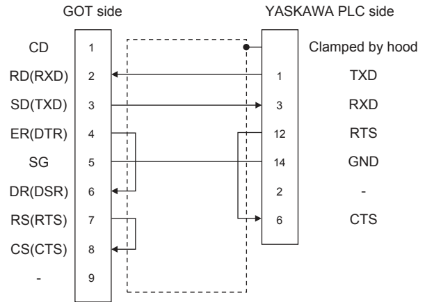
(d) RS-232 connection diagram 4)
