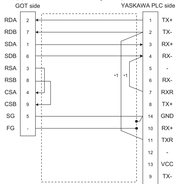
(d) RS-422 connection diagram 4)
