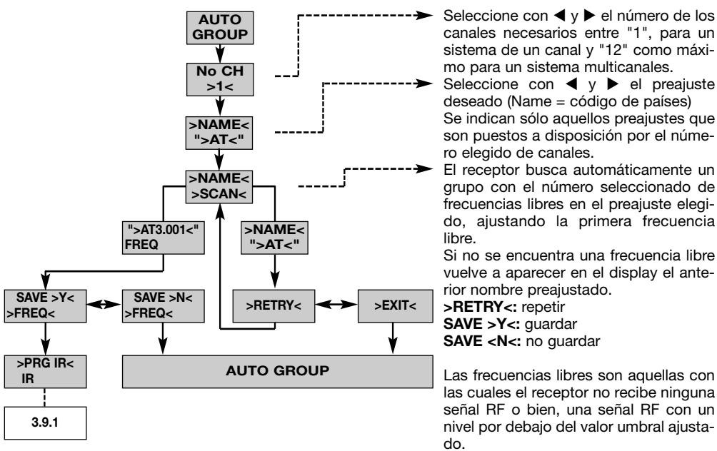
Diagrama 3: Búsqueda automática de un grupo de frecuencias anti-parasitarias
