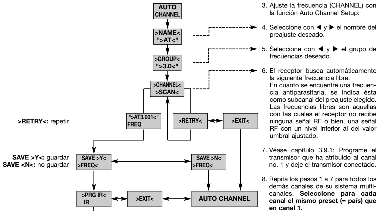
Diagrama 10: Búsqueda automática de frecuencias antiparasitarias para sistemas multicanales
