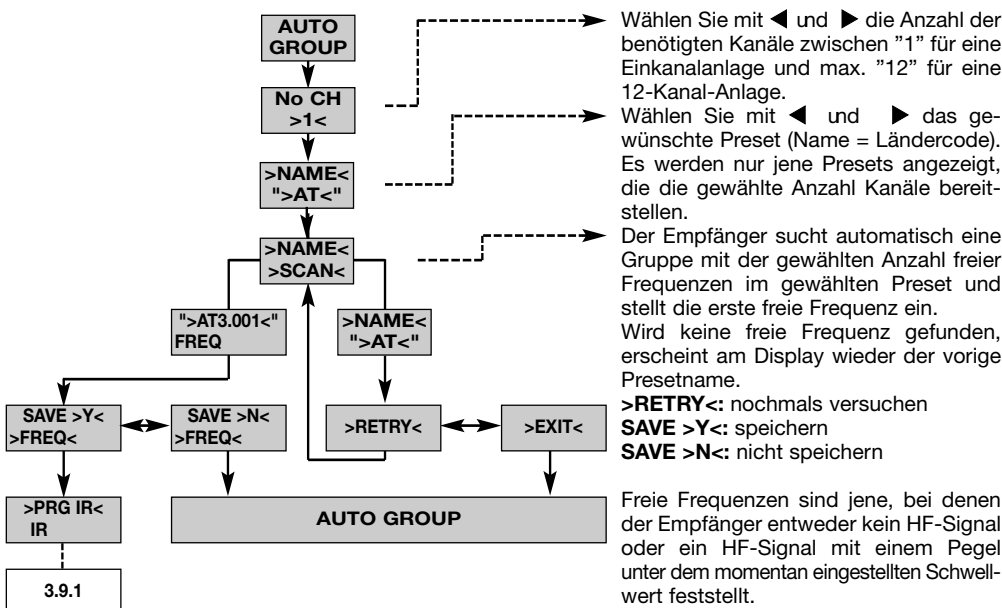
Diagramm 3: Automatische Suche nach einer störungsfreien Frequenzgruppe
