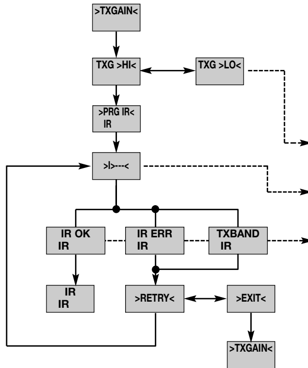
Diagramm 7: Eingangsempfindlichkeit des Handsenders einstellen
