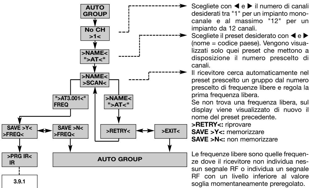
Diagramma 3: Ricerca automatica di un gruppo di frequenze esente da disturbi
