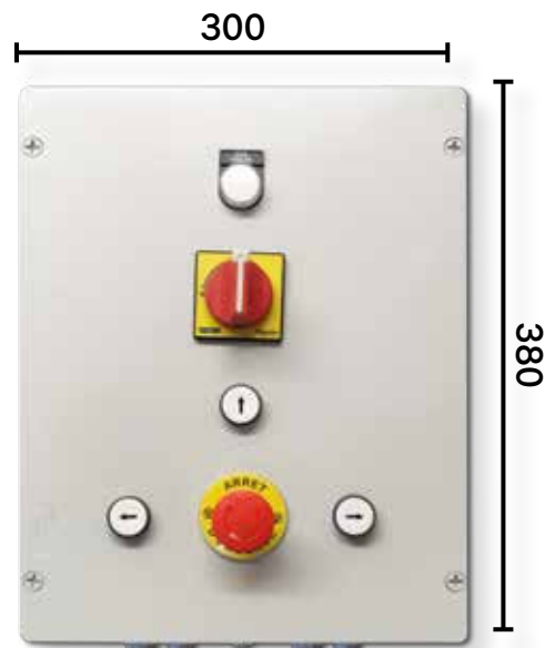
FTXNIV5B
