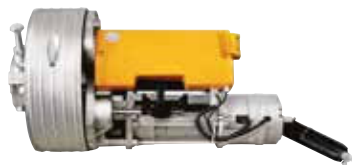
Moteur EASY 60 EP 145 Nm Avec frein et parachute Code : FAD6445P
