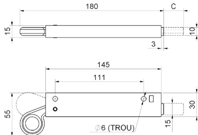
Verrou mécanique vertical À souder Existe en Inox acier inoxydable
