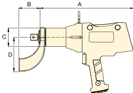
ETW-torque wrench
