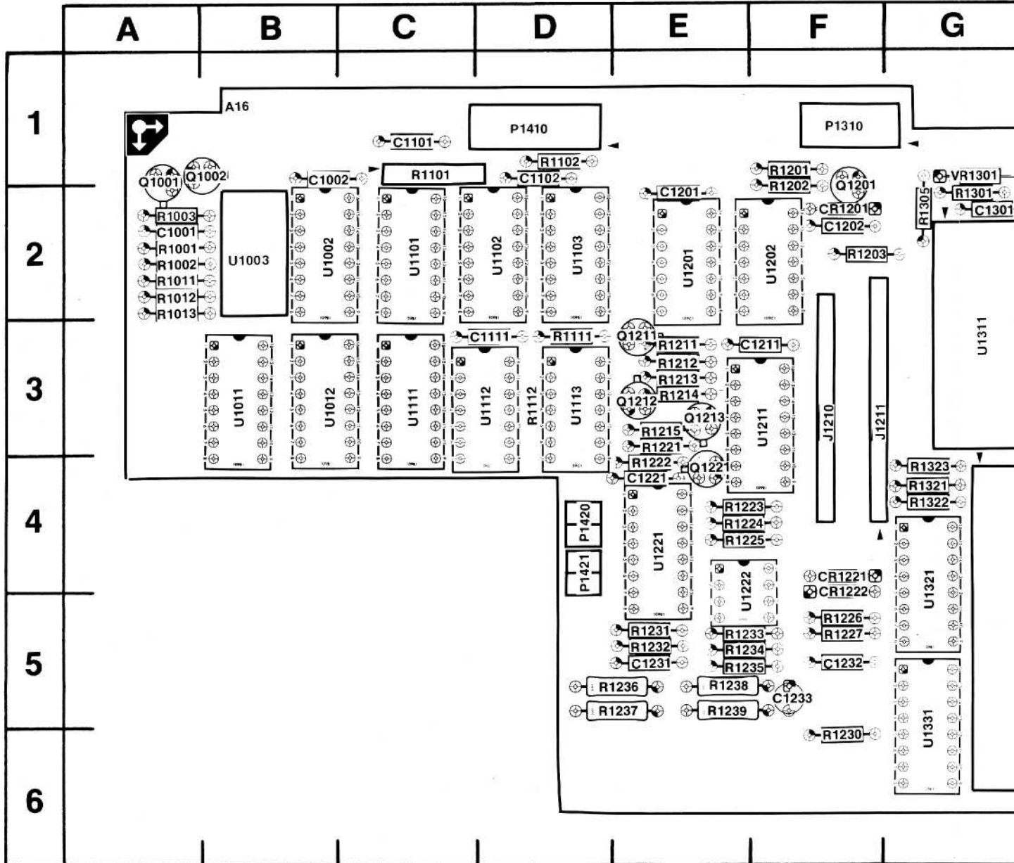
Fig. 8-9. Digital board
