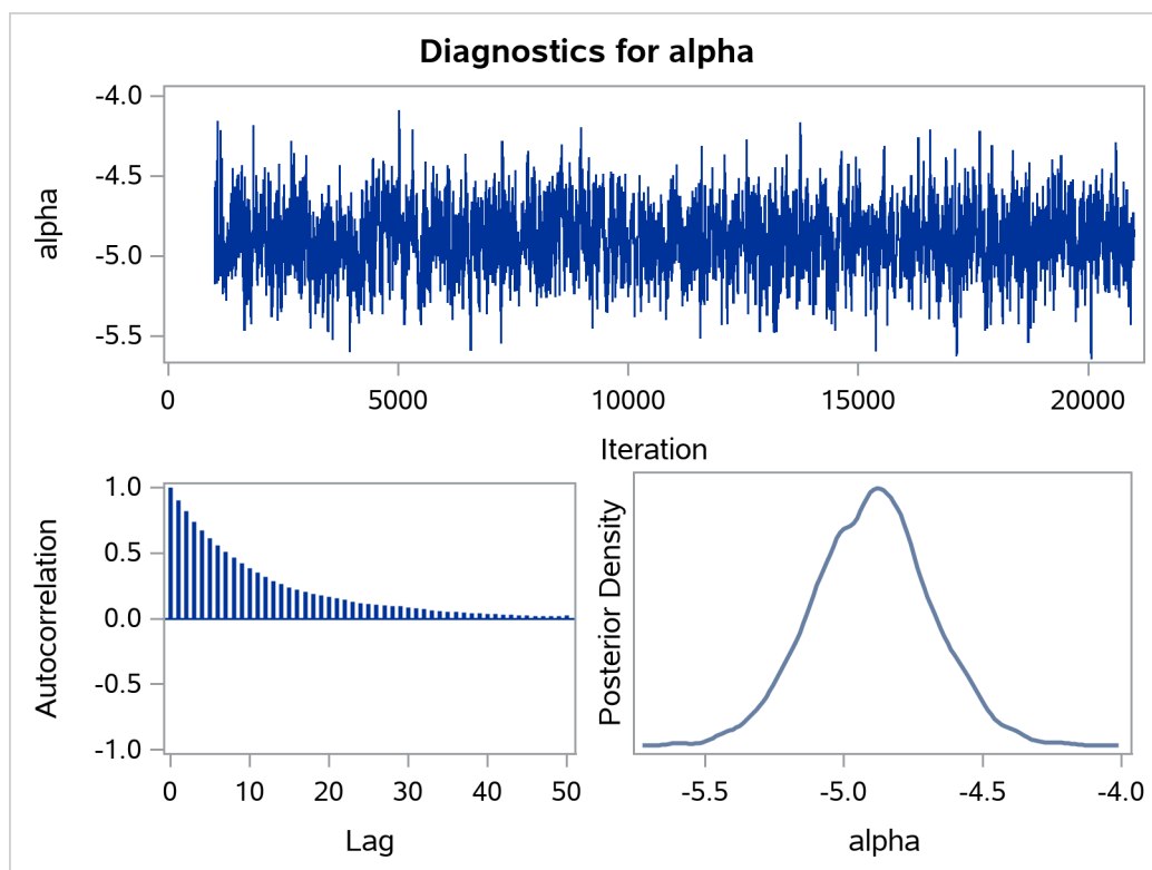
Output 77.6.1 Plots for Parameters
