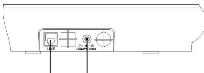
Conector del teléfono Conector del adaptador
