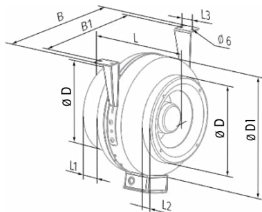
Centro-M 100 - Centro-M 315
