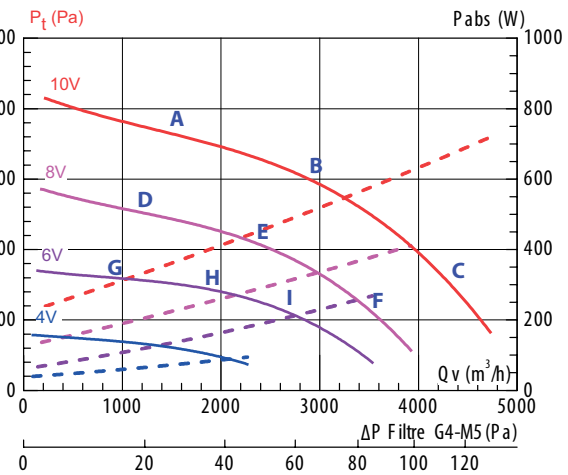
CMM EC 500
