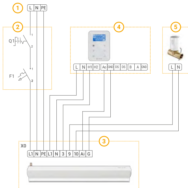
Version avec moteur EC
