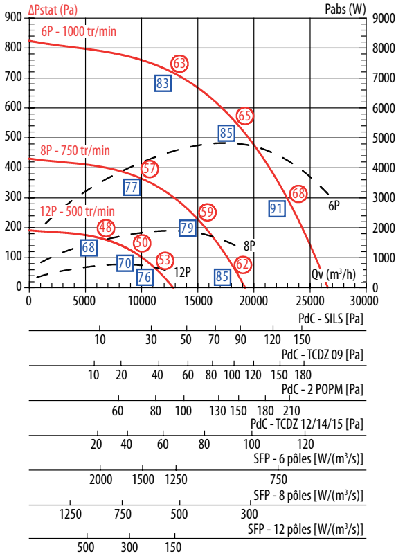
TEDH F400 800B TEDV F400 800B
