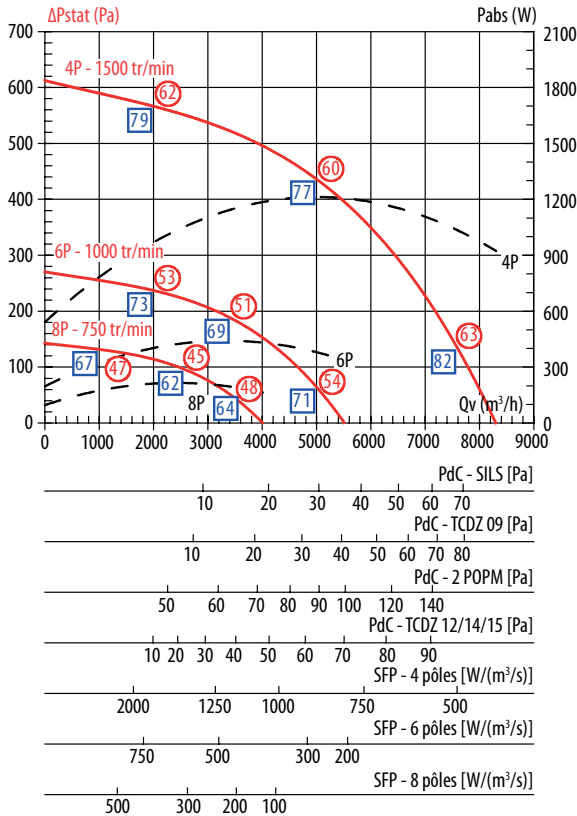
TEDH F400 450 TEDV F400 450
