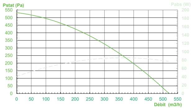
CMM 125 EC
