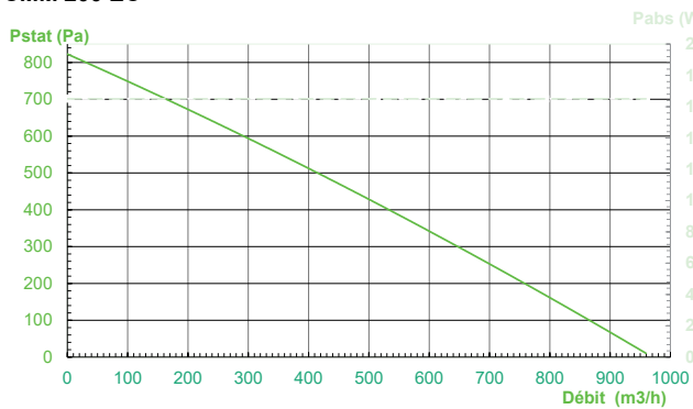
CMM 200 EC
