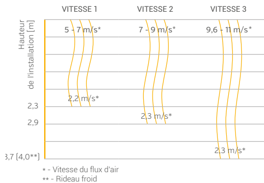
Volume vertical du flux d'air (hauteur maximale de l'installation)
