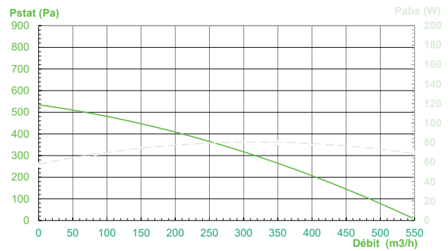
CMM 160 EC
