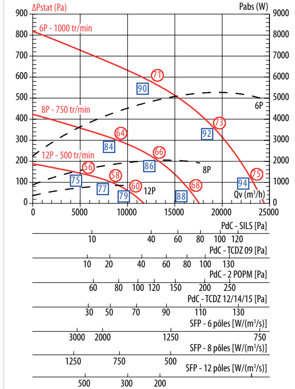
TEDH F400 810 TEDV F400 810
