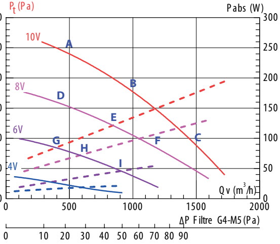
CMM EC 355
