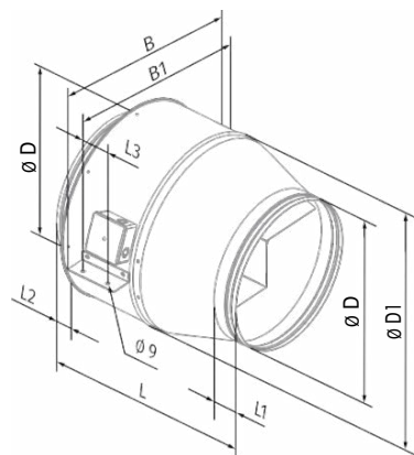
Centro-M 355 - Centro-M 450
