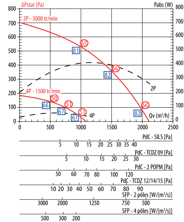
TEDH F400 250 TEDV F400 250
