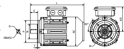
B14
