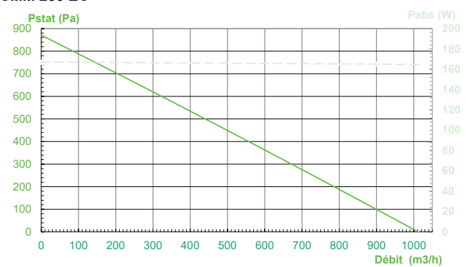
CMM 250 EC
