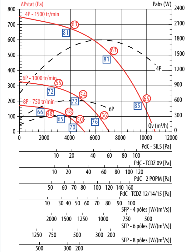
TEDH F400 500 TEDV F400 500
