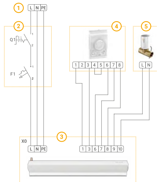
Version avec moteur AC
