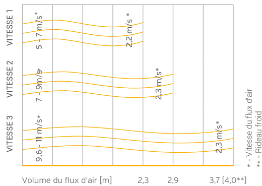
Volume horizontal du flux d'air (relatif à l'installation verticale)
