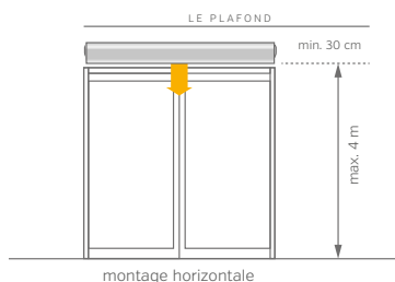
montage horizontale
