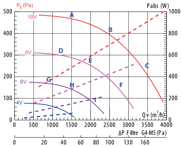
CMM EC 450
