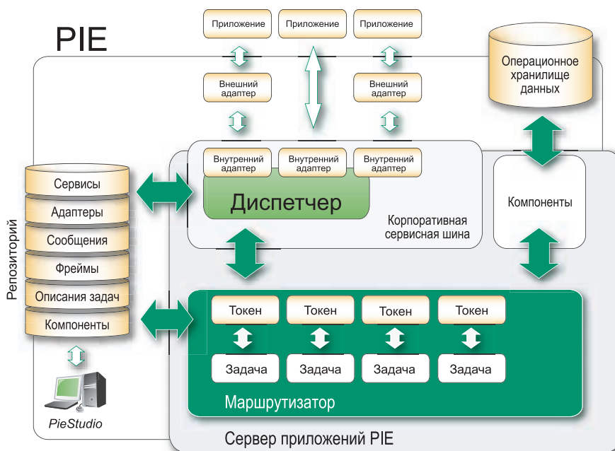
Схема взаимодействия интеграционной платформы СМА PIE и IT-инфраструктуры предприятия
