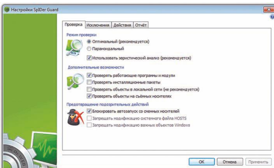
Рис. 1. Настройки SpIDer Guard
