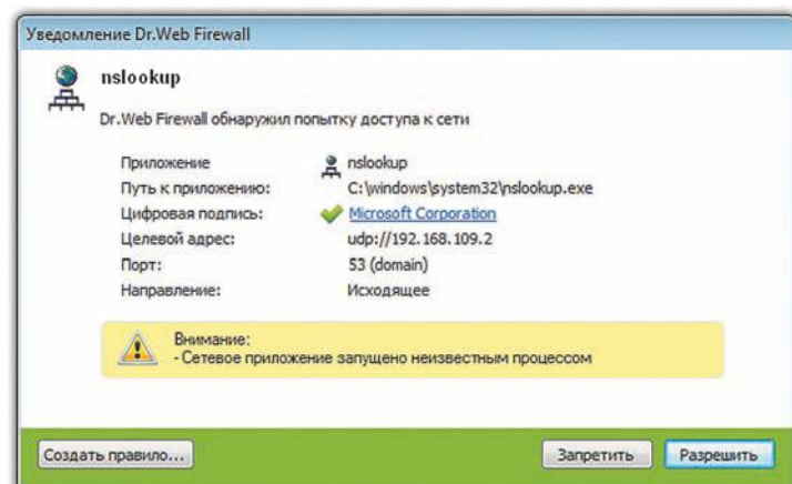
Рис. 2. Уведомление брандмауэра Dr.Web
