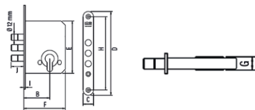
Wymiary (mm)
