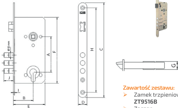
Wymiary (mm)
