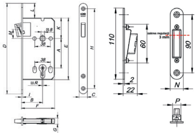
Wymiary (mm)
