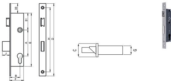
Wymiary (mm)
