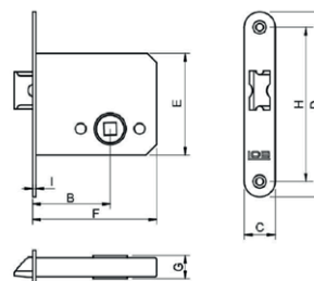
Wymiary (mm)
