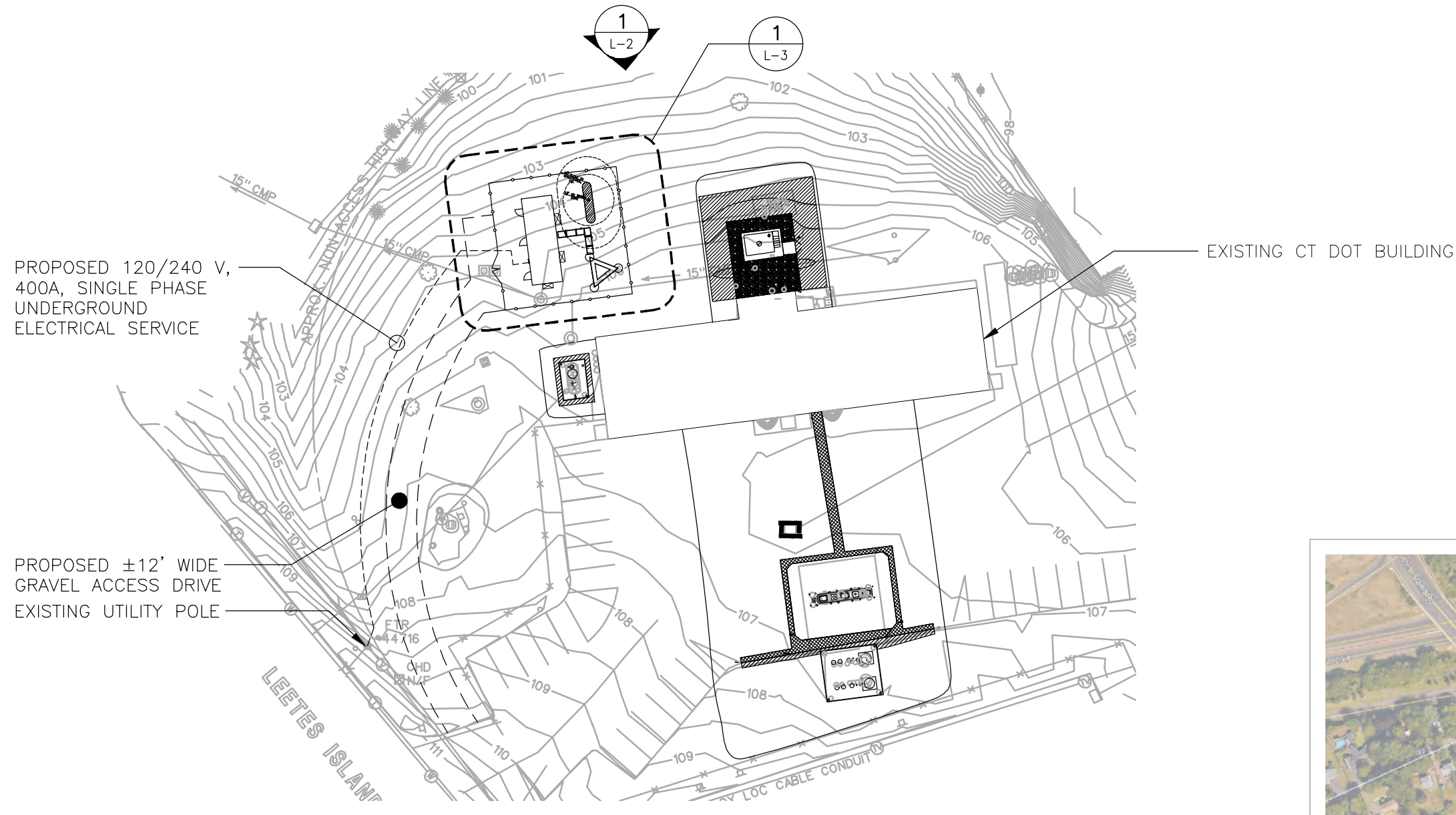
1 L-1 SITE PLAN SCALE: 1" = 50'
