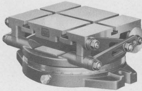
TAFT-PEIRCE STYLE 9175
