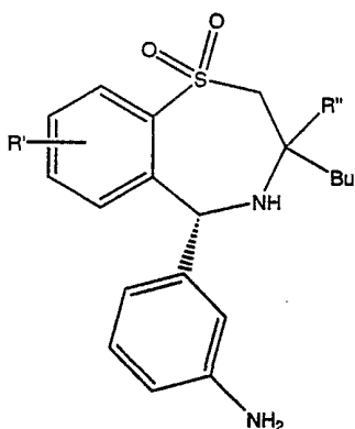
44, R' = 3,4-acetonide, R'' = Et 45, R' = 4-(dimethylamino), R'' = Et 46, R' = 3,4-acetonide, R'' = Bu 47, R' = 4-(dimethylamino), R'' = Bu
