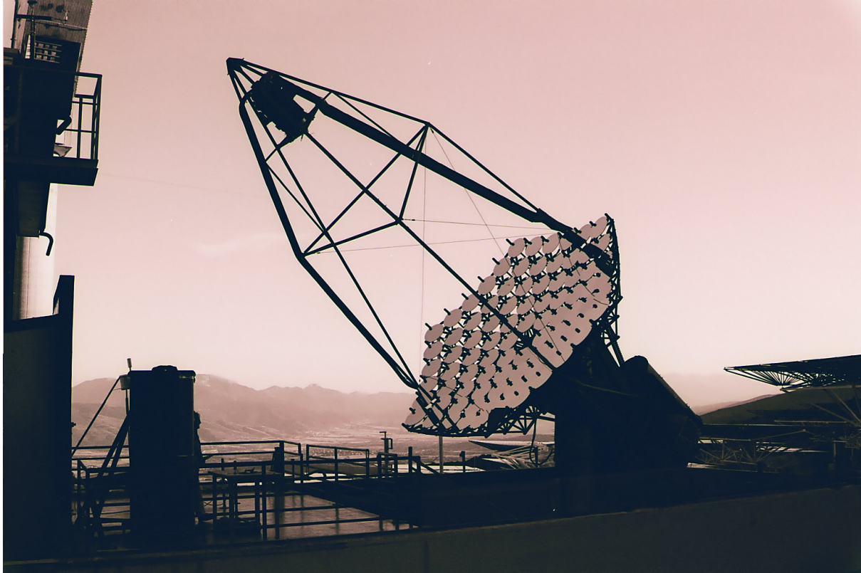
FIG. 3.2: L'imageur CAT photographié juste avant le coucher de Soleil, qui envoie encore ses rayons sur la tour (visible dans la partie gauche de la photo). Le hangar est ouvert, le télescope est en élévation au dessus de sa position de repos. On voit bien le réflecteur composé de 90 miroirs individuels, et la caméra dans son plan focal.
