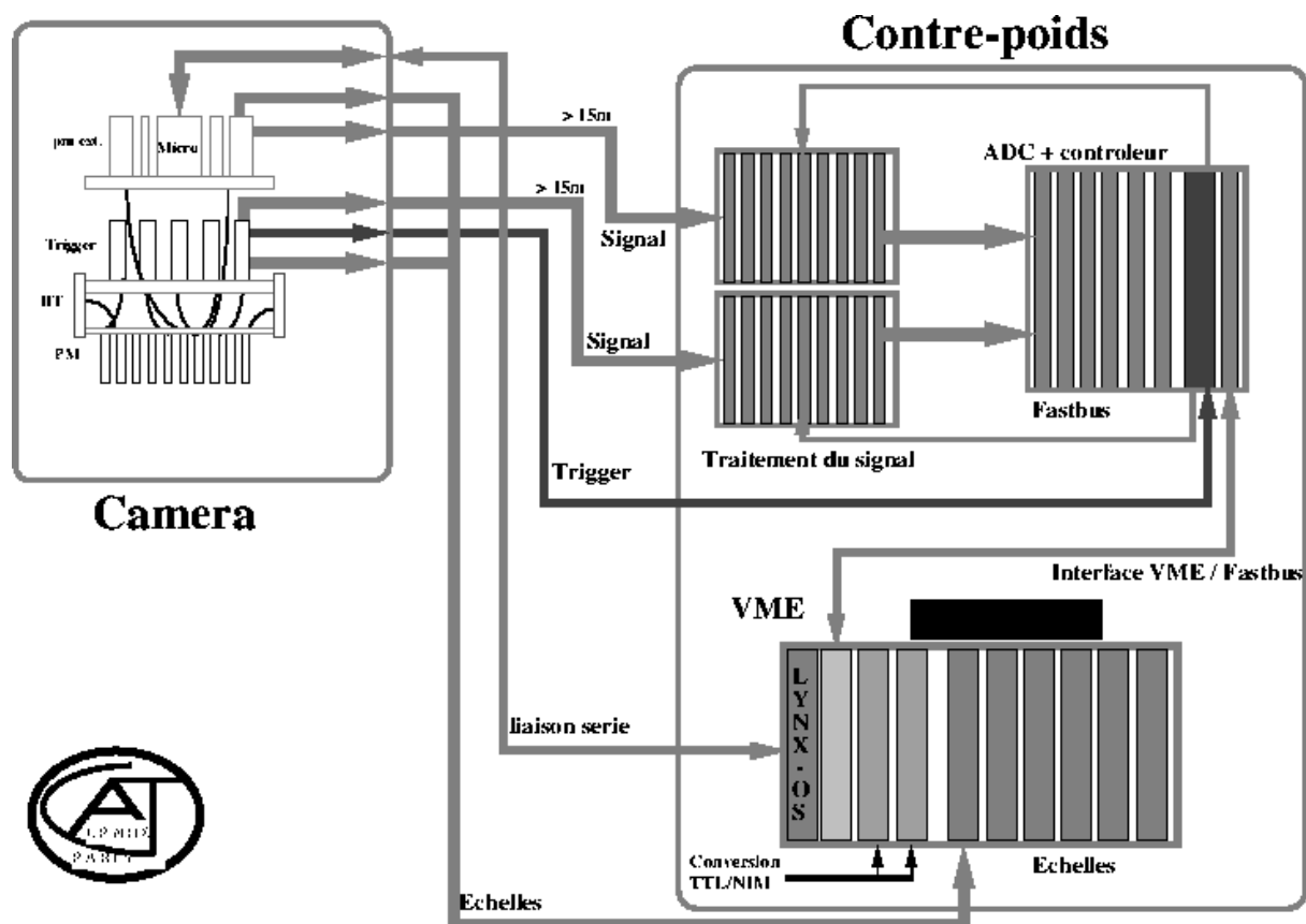
FIG. 3.4: Schéma de répartition de l'électronique du détecteur. La partie compacte, située dans la caméra, inclut la logique de déclenchement. La deuxième partie, placée dans le contrepois du télescope, contient les alimentations de haute et de basse tension, ainsi que l'électronique de traitement analogique des signaux.
