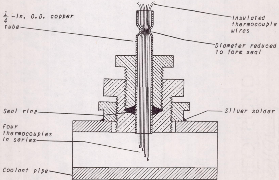
(d) Coolant thermocouples in coolant pipes.
