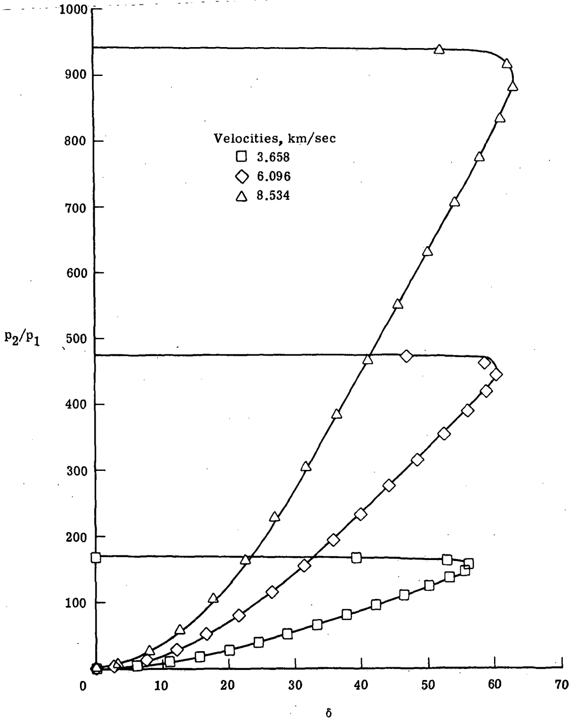
(g) p_2/p_1 .
