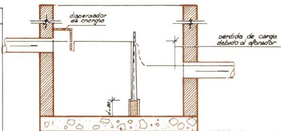
CORTE LONGITUDINAL
