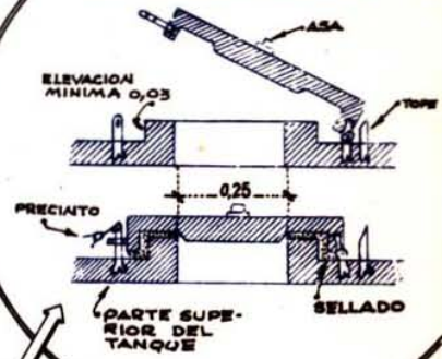
CARACTERÍSTICAS DE LAS TAPAS SUPERIORES
