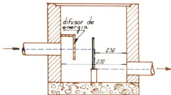
CORTE LONGITUDINAL
