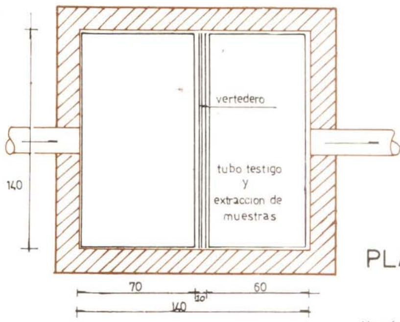
CORTE LONGITUDINAL
