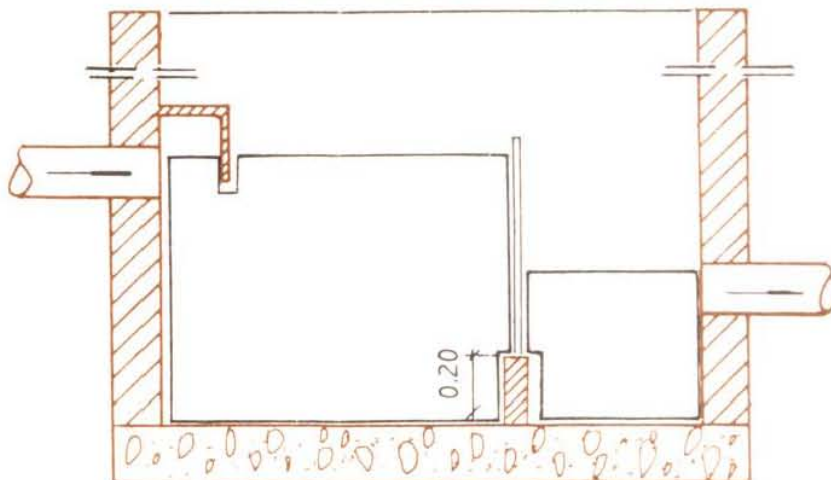
CORTE LONGITUDINAL
