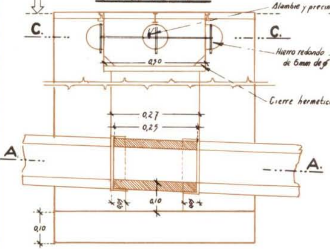
CORTE POR B-B
