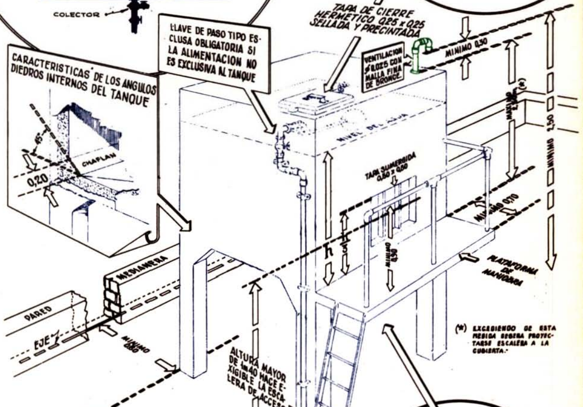
TANQUE PARA CAPACIDADES DESDE 4.000 L e DIVIDIDO
