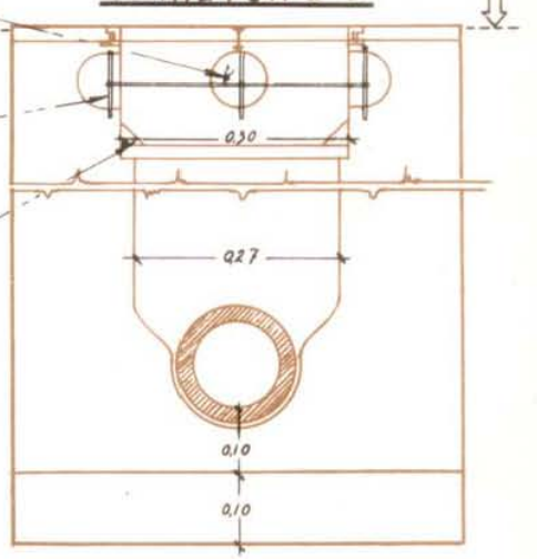
CORTE POR D-D
