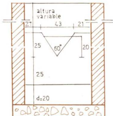
CORTE TRANSVERSAL
