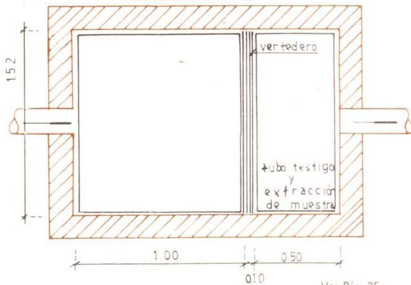
PLANTA
