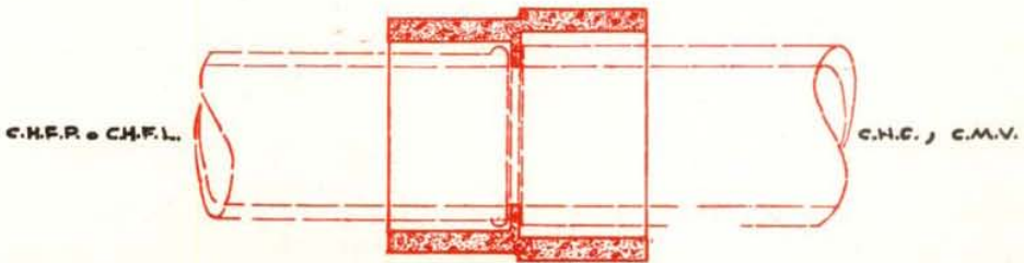
DETALLE DEL ANILLO ESPECIAL DE HORMIGON
