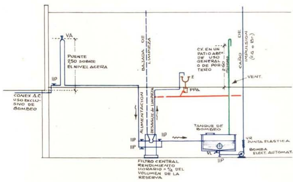
VARIANTE: EQUIPO DE 3 BOMBAS CON DOBLE CAÑERIA DE IMPULSION.
