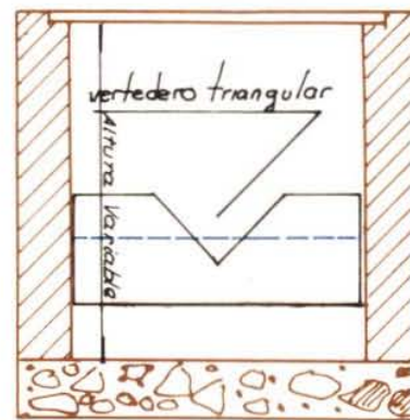
CORTE TRANSVERSAL
