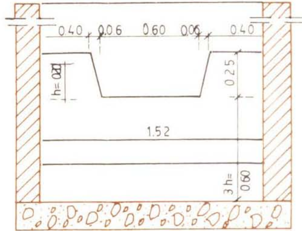
CORTE LONGITUDINAL
