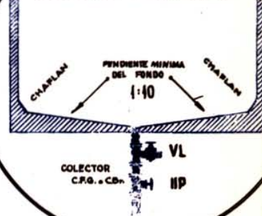
CARACTERÍSTICAS DEL FONDO Y DEL COLECTOR
