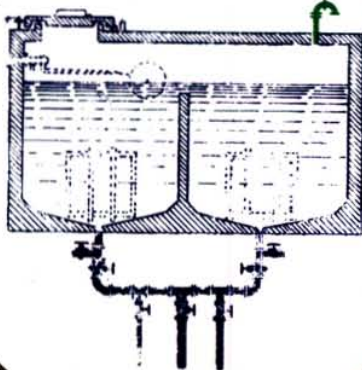
TANQUE PARA CAPACIDADES DESDE 4.000 L e DIVIDIDO
