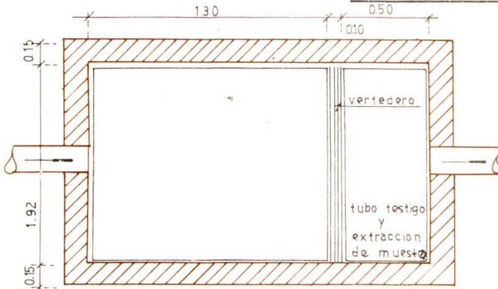
PLANTA
