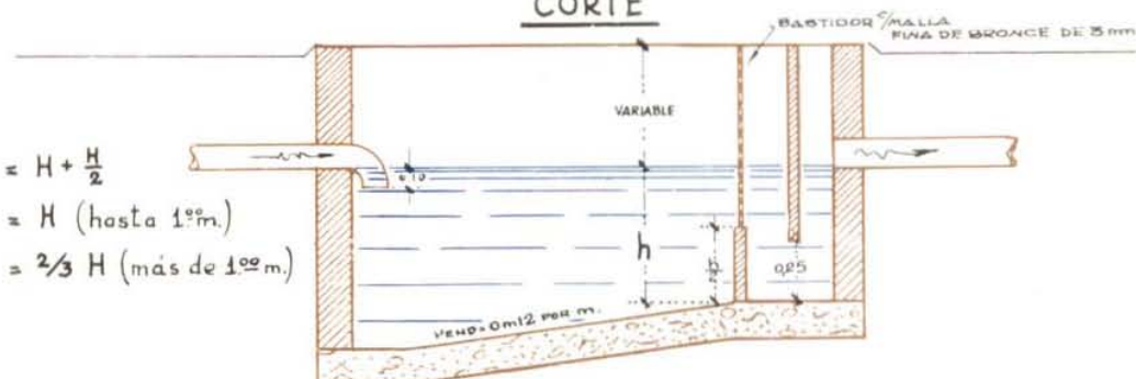
CORTE
