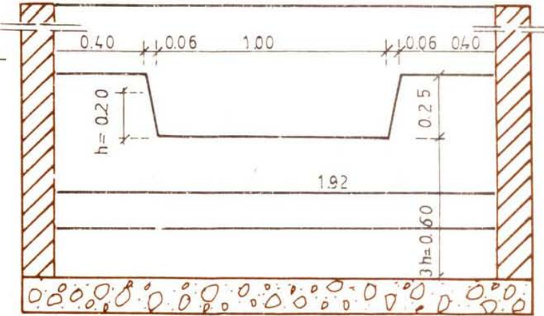
CORTE TRANSVERSAL
