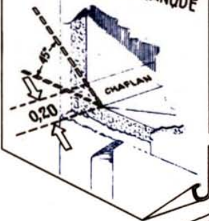
CARACTERÍSTICAS DE LOS ANGULOS DIEDROS INTERNOS DEL TANQUE
