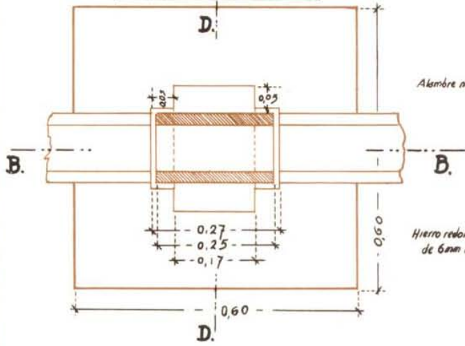
PLANTA POR A-A
