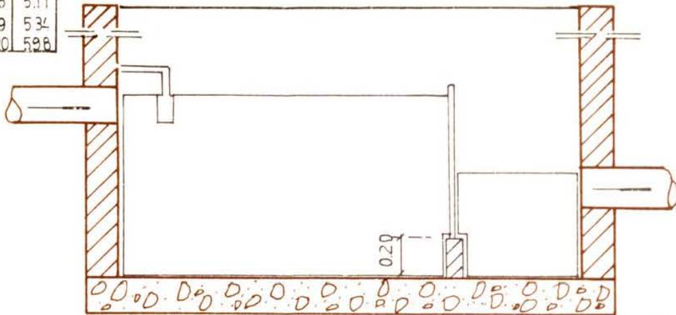
CORTE LONGITUDINAL
