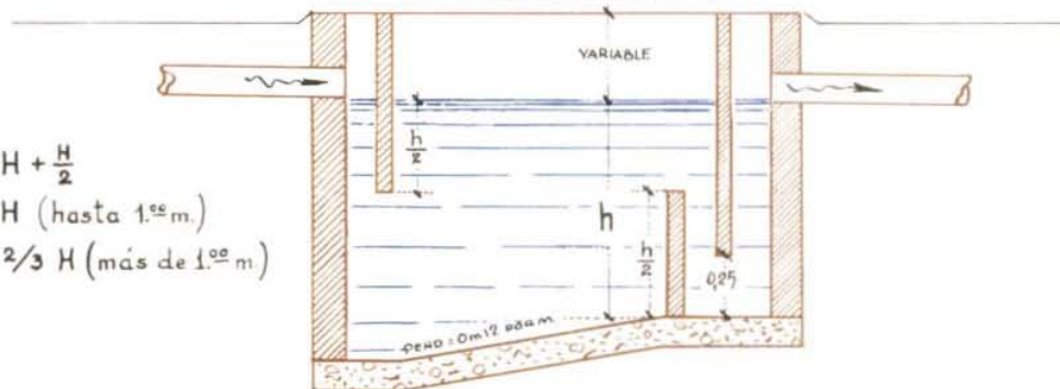
CORTE
