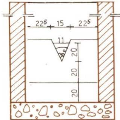
CORTE TRANSVERSAL
