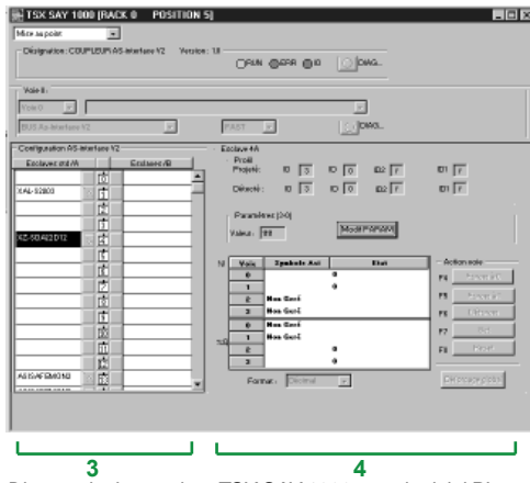
Diagnostic du coupleur TSX SAY 1000 sous logiciel PL7
