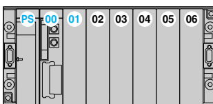
Rack principal adresse 0 avec alimentation et processeur simple format
