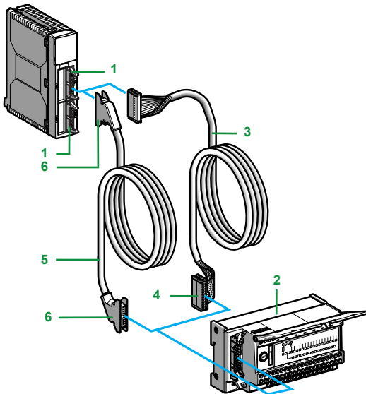
Nappe et câble de raccordement
