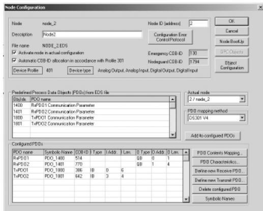
Exemple d'écran SyCon de configuration des équipements
