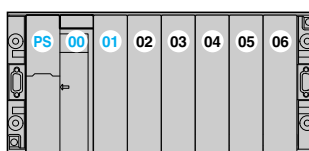
Rack extension adresse n avec alimentation double format
