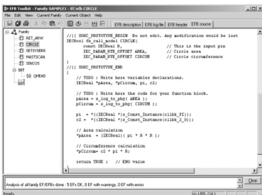
EFB Toolkit : Editeur
