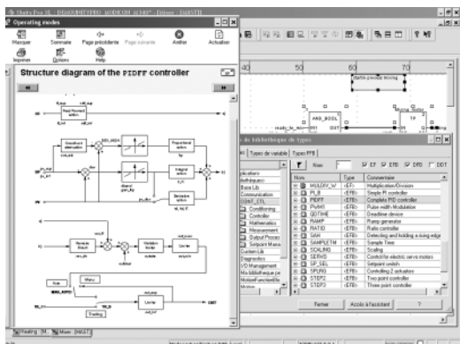
CONT_CTL, la régulation programmable intégrée dans Unity Pro
