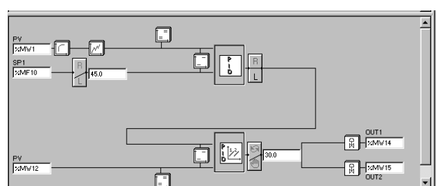
Boucle cascade
