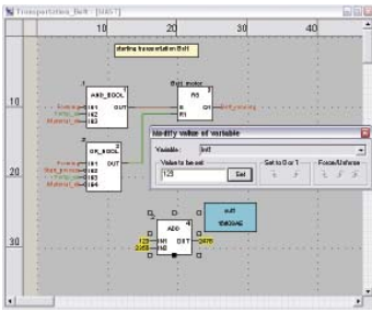
Animation dynamique/réglage
