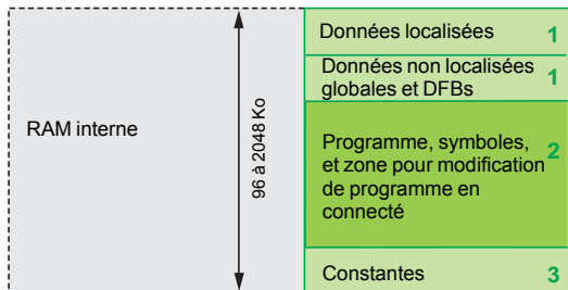
Processeur sans carte mémoire PCMCIA
