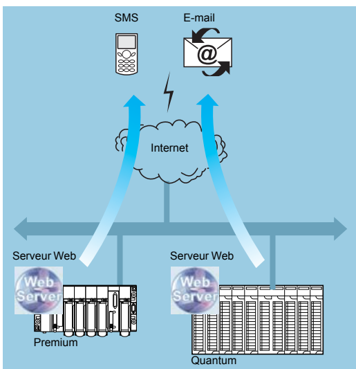
Envoi d'E-mail
