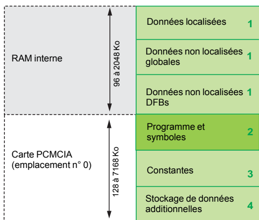
Processeur avec carte mémoire PCMCIA à l'emplacement n° 0
