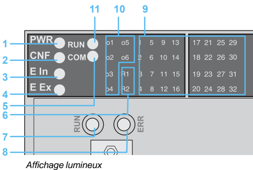
Affichage lumineux
