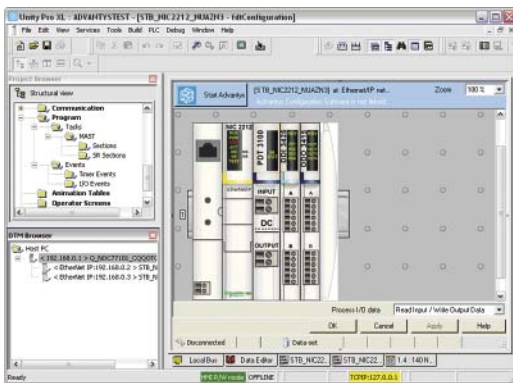
Editeur DTM (îlot Modicon STB)
