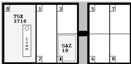
Déclaration du module maître TSX Micro TSX SAZ 10
