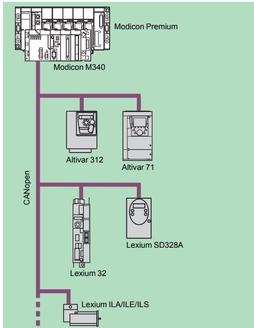
MFB : La commande de mouvement distribuée sur CANopen
