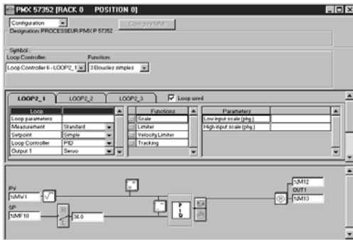
Configuration des voies de régulation
