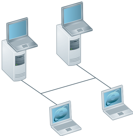
Architecture redondante avec 2 Control Client sur serveurs et 2 Web View Only Client
