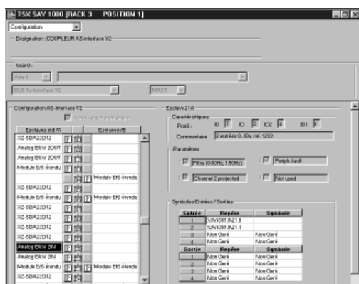
Configuration des équipements esclaves AS-Interface dans le module Premium TSX SAY 1000
