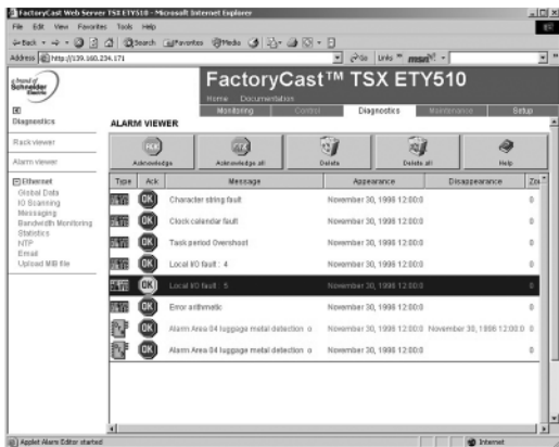
Visualisation d'alarmes
