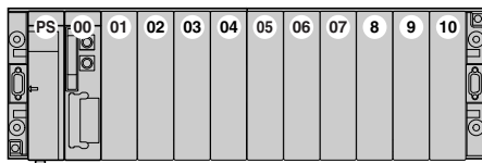
Rack adresse n (exemple avec 1 rack 12 emplacements, alimentation et processeur simple format)
