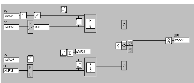
Boucle auto-sélective
