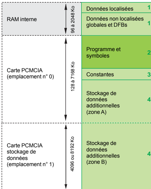
Processeur avec cartes mémoire de type mixte à l'emplacement n°0 et de type stockage de données à l'emplacement n° 1 (1)
