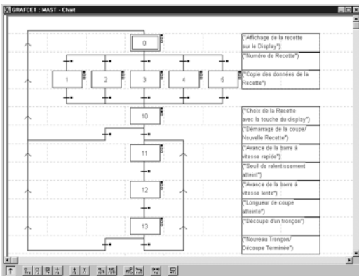
Editeur graphique langage Grafcet SFC
