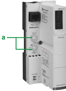
Module réseau NIM des E/S Modicon STB
