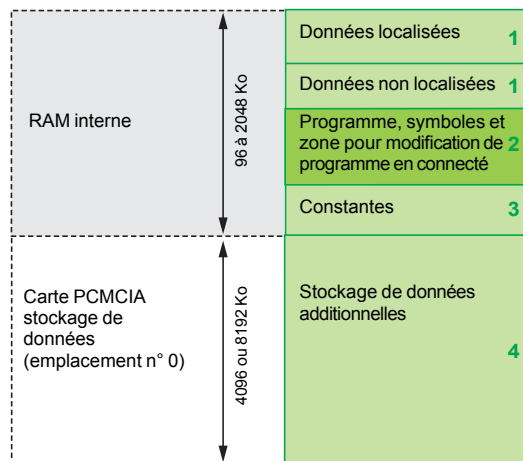
Processeur avec carte mémoire de type stockage de données à l'emplacement n° 0
