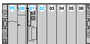
Rack principal adresse 0 avec alimentation double format et processeur simple format
