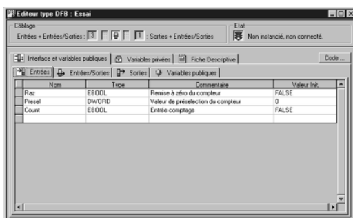
Editeur type DFB
