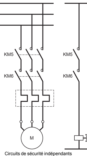
Circuits de sécurité indépendants
