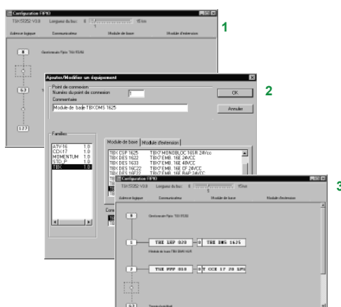
Configuration du bus Fipio
