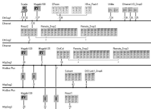
Configuration de l'automatisation multi-stations
