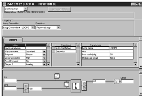
Configuration d'une boucle process
