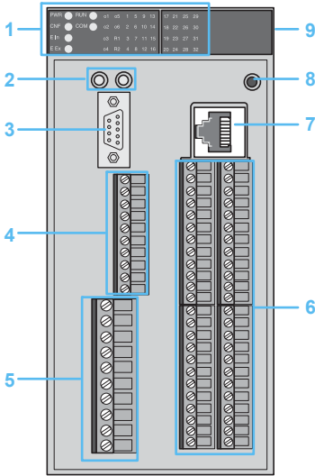
Contrôleur configurable XPS MC, avec connecteurs à vis
