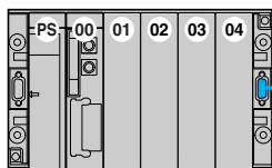
Rack adresse n, exemple avec 2 racks 6 emplacements, alimentations et processeur simple format
