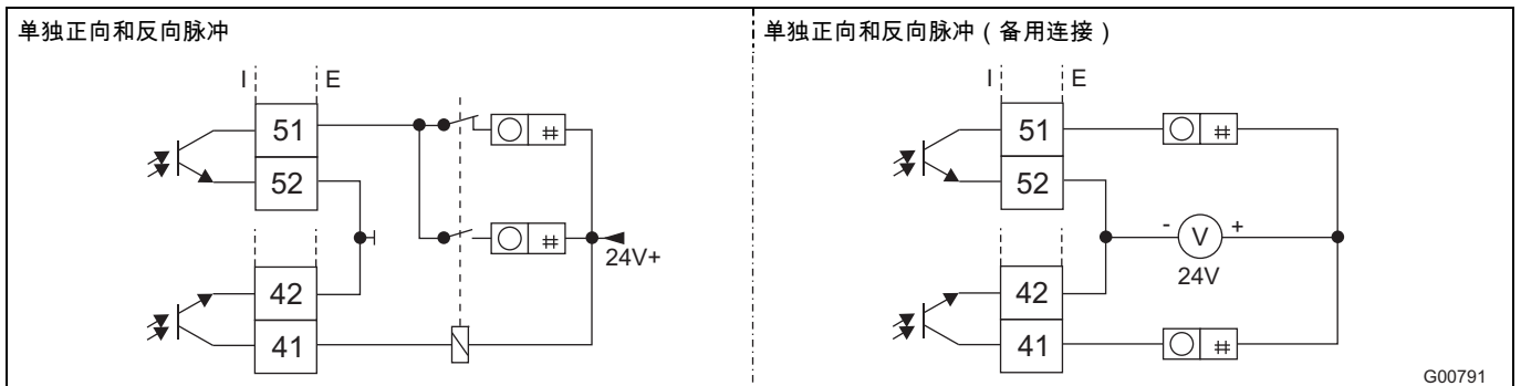
图 45 : ( I = 内部, E = 外部)
