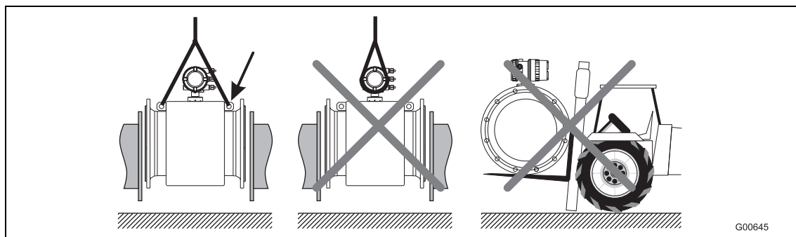
图 4 : DN 400 以上尺寸法兰连接设备的运输
