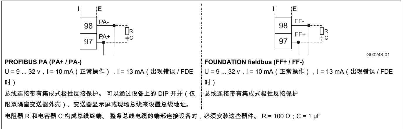
图 43 : ( I = 内部, E = 外部)
