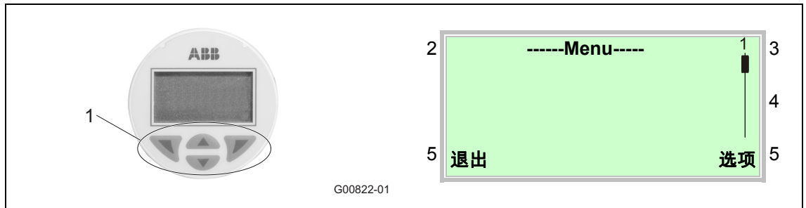
图 47： LCD 指示灯
