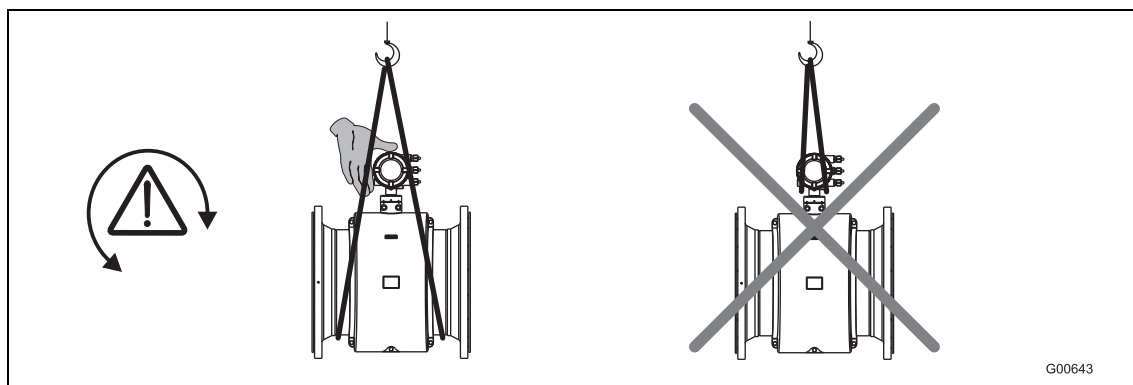
图 3 : DN 450 以下尺寸法兰连接设备的运输
