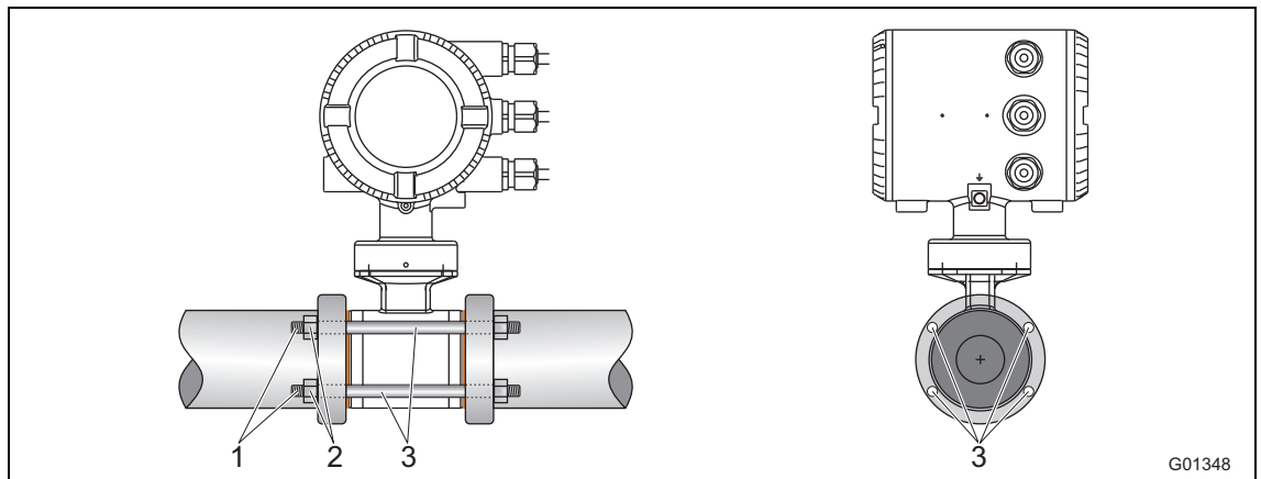
图 6： 对夹式安装套件
