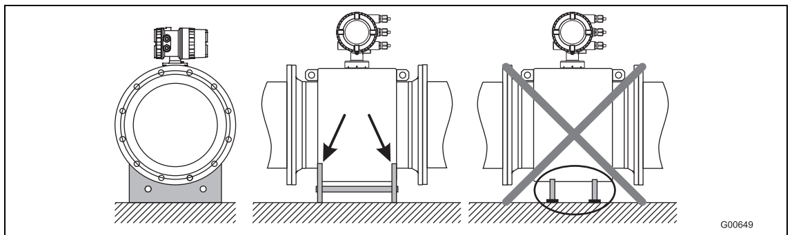
图 5：DN 400 以上尺寸的流量计的支撑件
