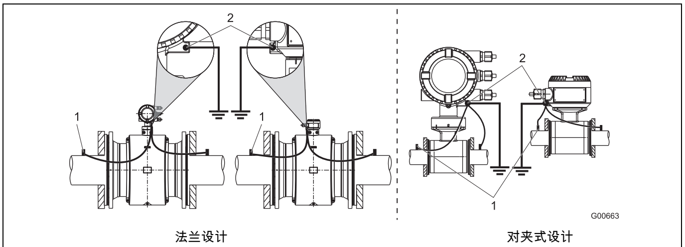
图 22： 金属管，不带内衬（示例）
