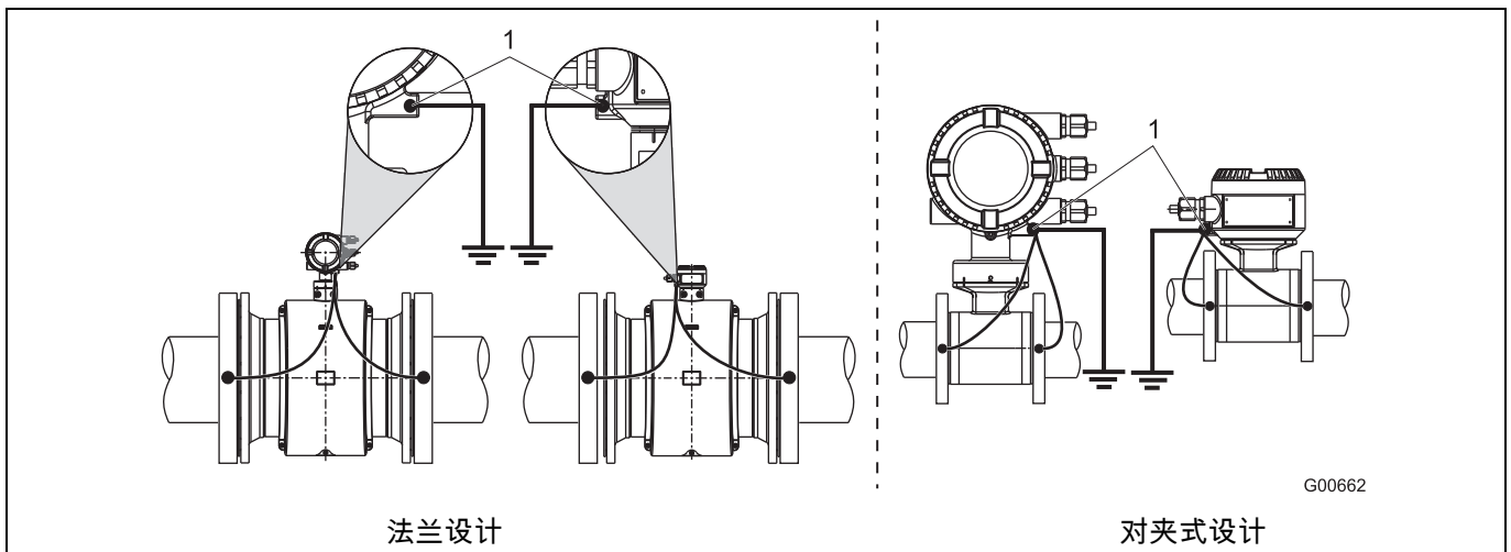
图 21： 金属管，不带内衬（示例）
