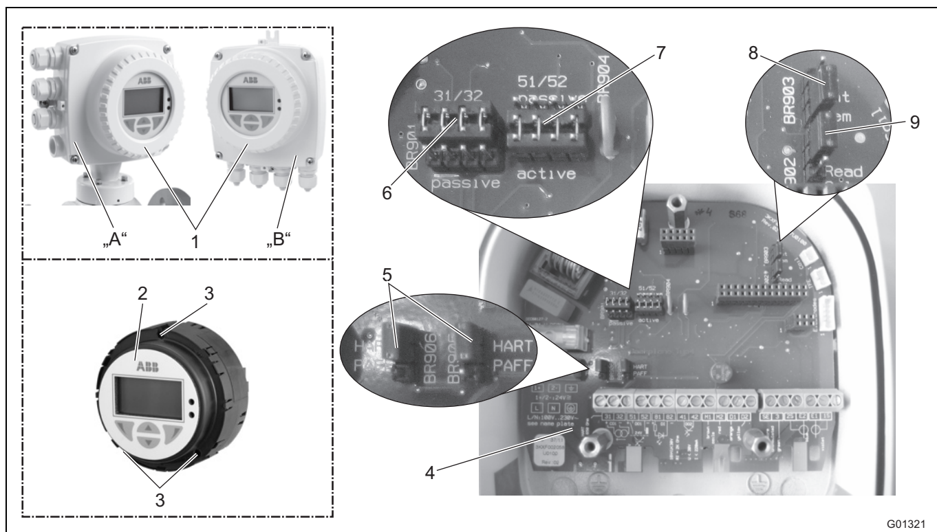
图 51： 单壳体中的跳线
