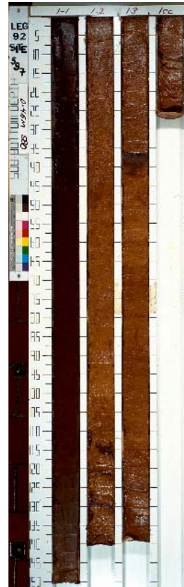
Core 92-597-1H
