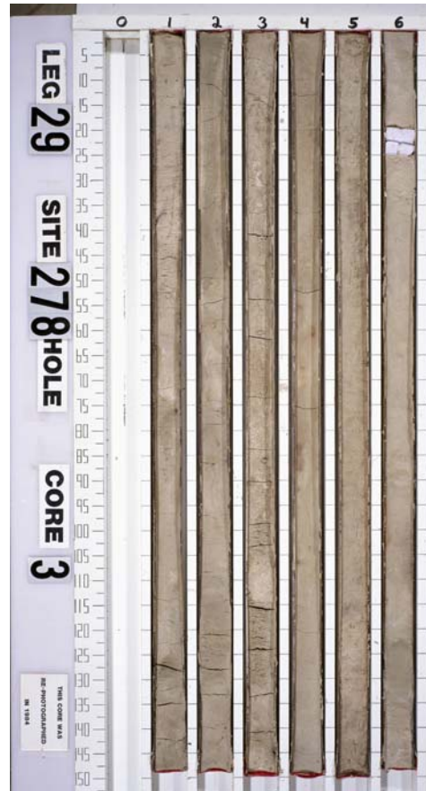
Core 29-278-3R
