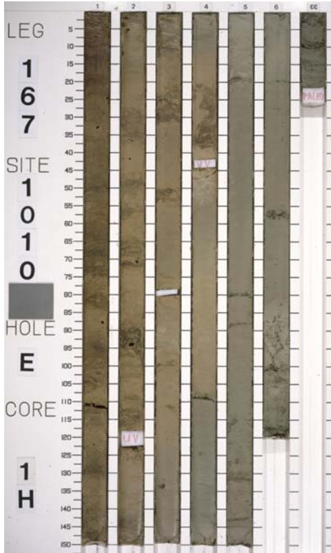
Core 167-1010E-1H
