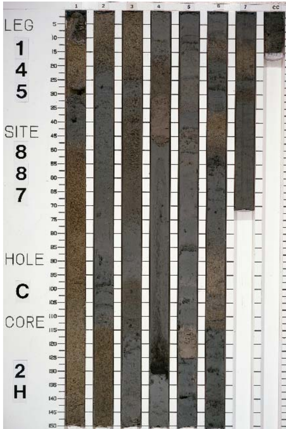
Core 145-887C-2H
