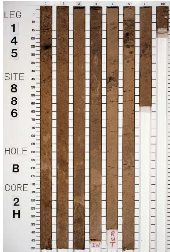
Core 145-886B-2H
