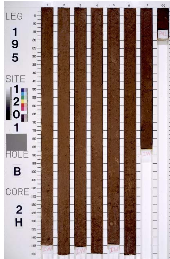
Core 195-1201B-2H
