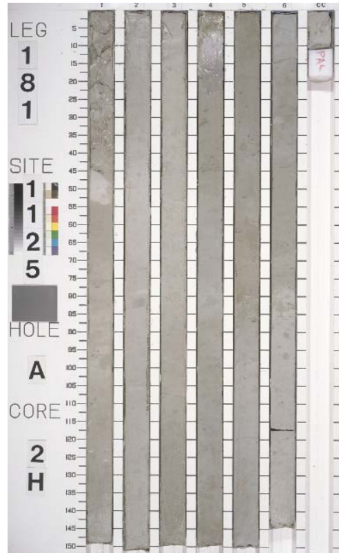
Core 181-1125A-2H
