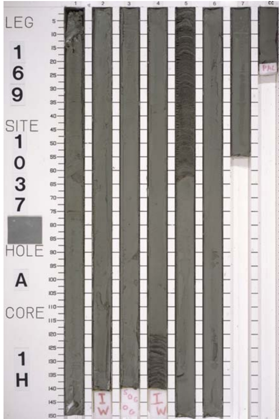
Core 169-1037A-1H
