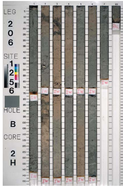
Core 206-1256B-2H
