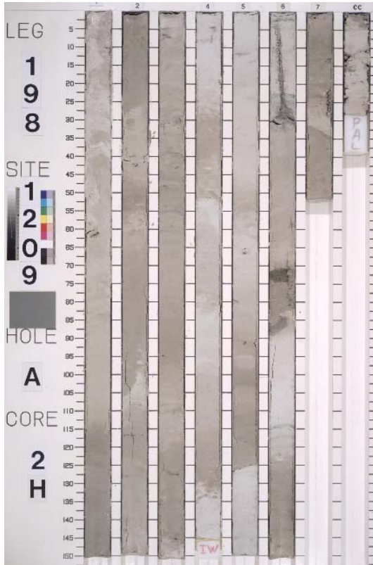
Core 198-1209A-2H
