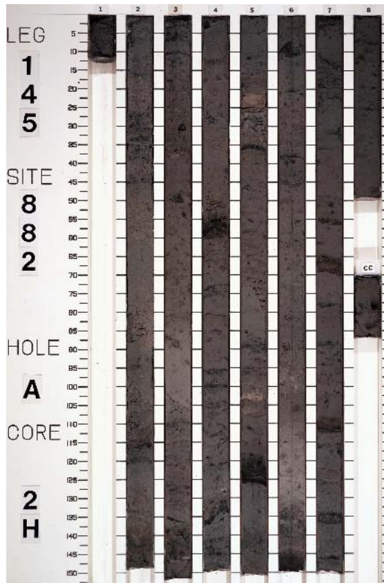
Core 145-882A-2H
