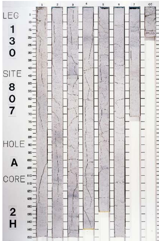
Core 130-807A-2H
