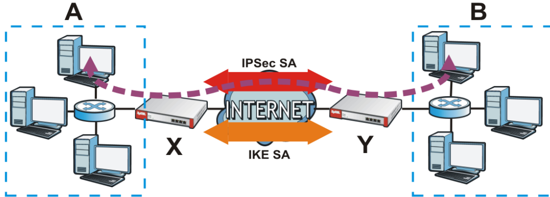
Figure 224 VPN: IKE SA and IPsec SA
