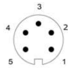
MINI Cable - Pin Out / Color Code (Male View)
