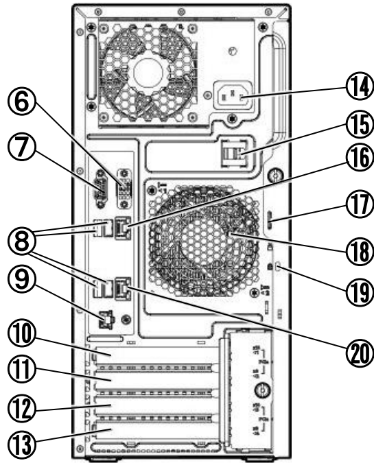
全モデル共通 背面図
