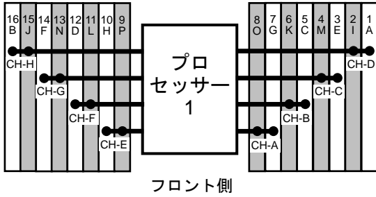
ProLiant DL325 Gen10 Plus v2 サーバーのプロセッサとメモリ スロットのレイアウト
