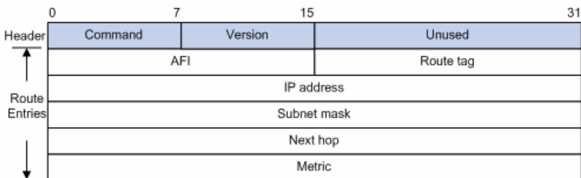
Figure 10-24 RIPv2 Message Format
