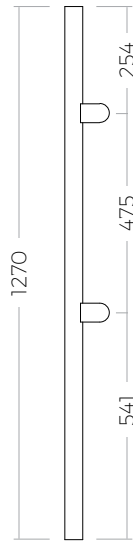
SSPPG166X42E End Post 42"
