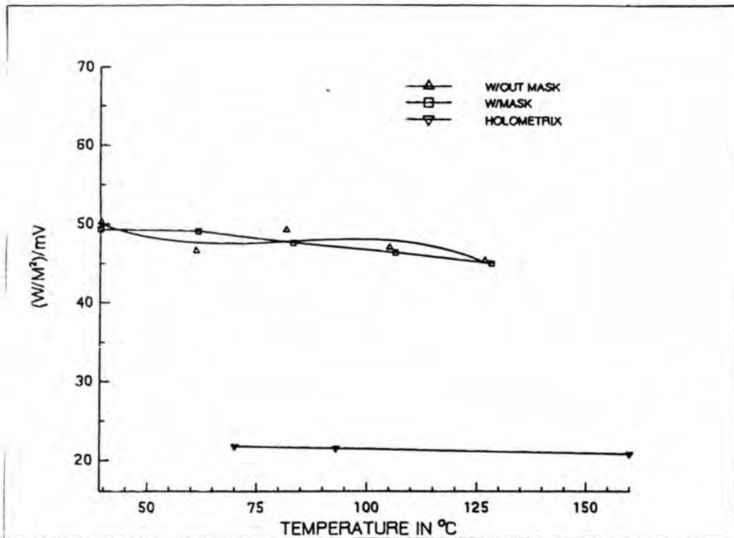
Figure 8. ITI #B-360 calibration curves.
