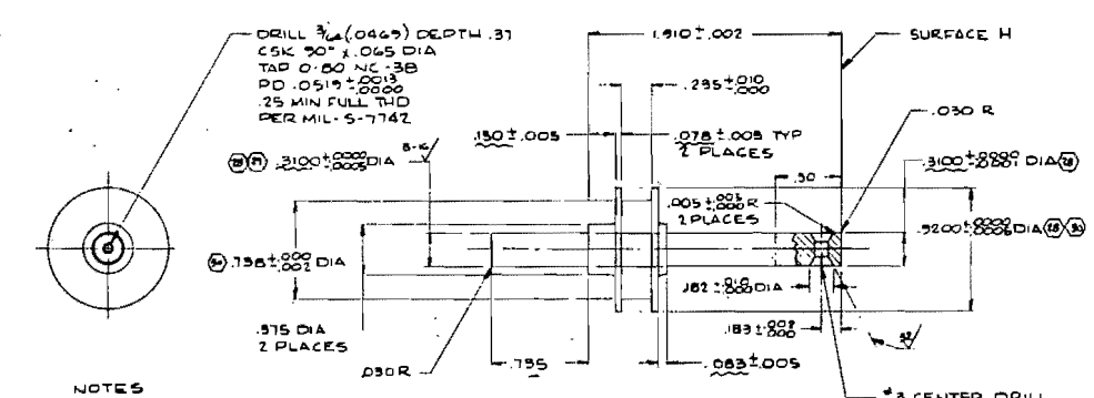
(49) PLUNGER
